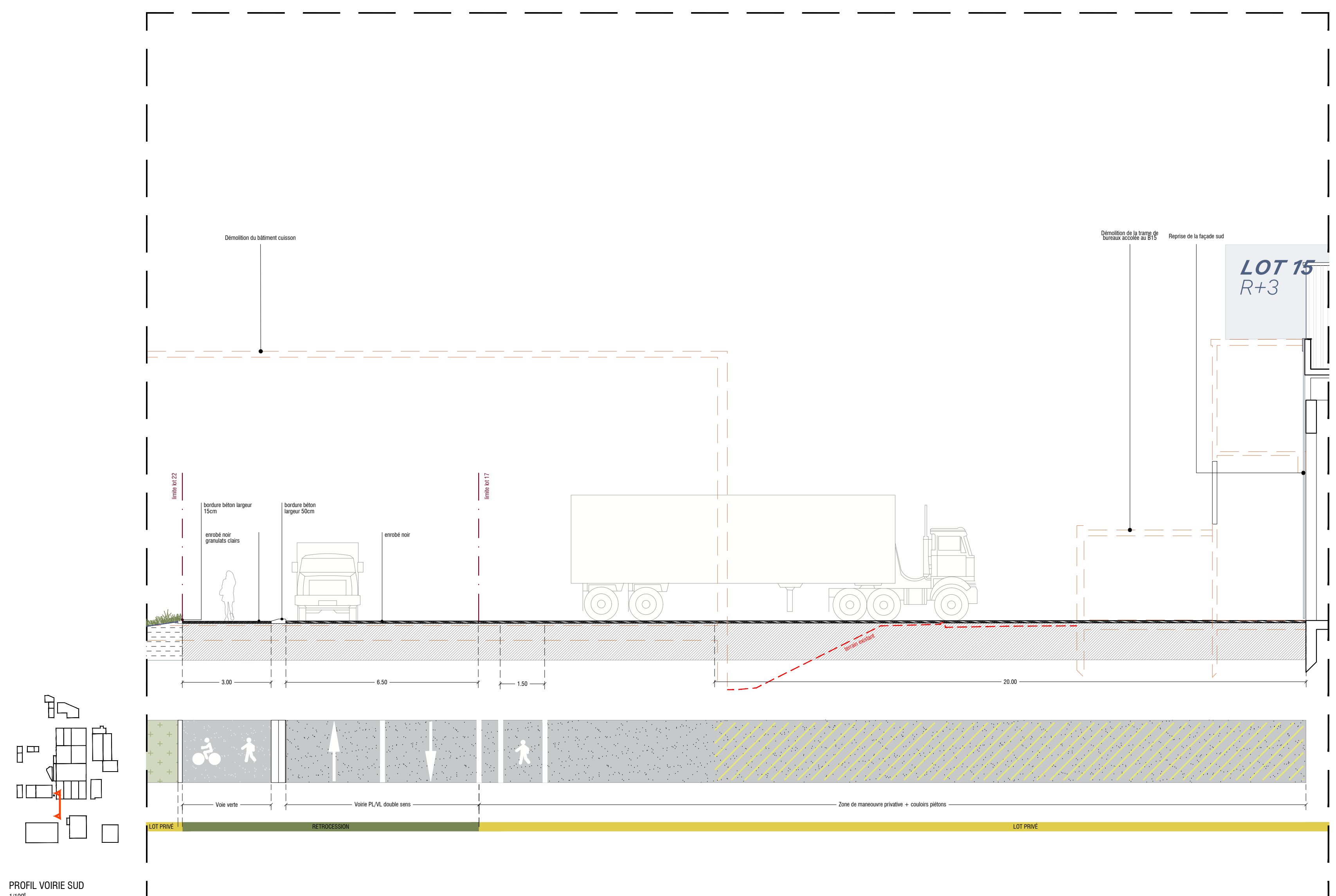
PROFIL VOIRIE SUD 1/100'
