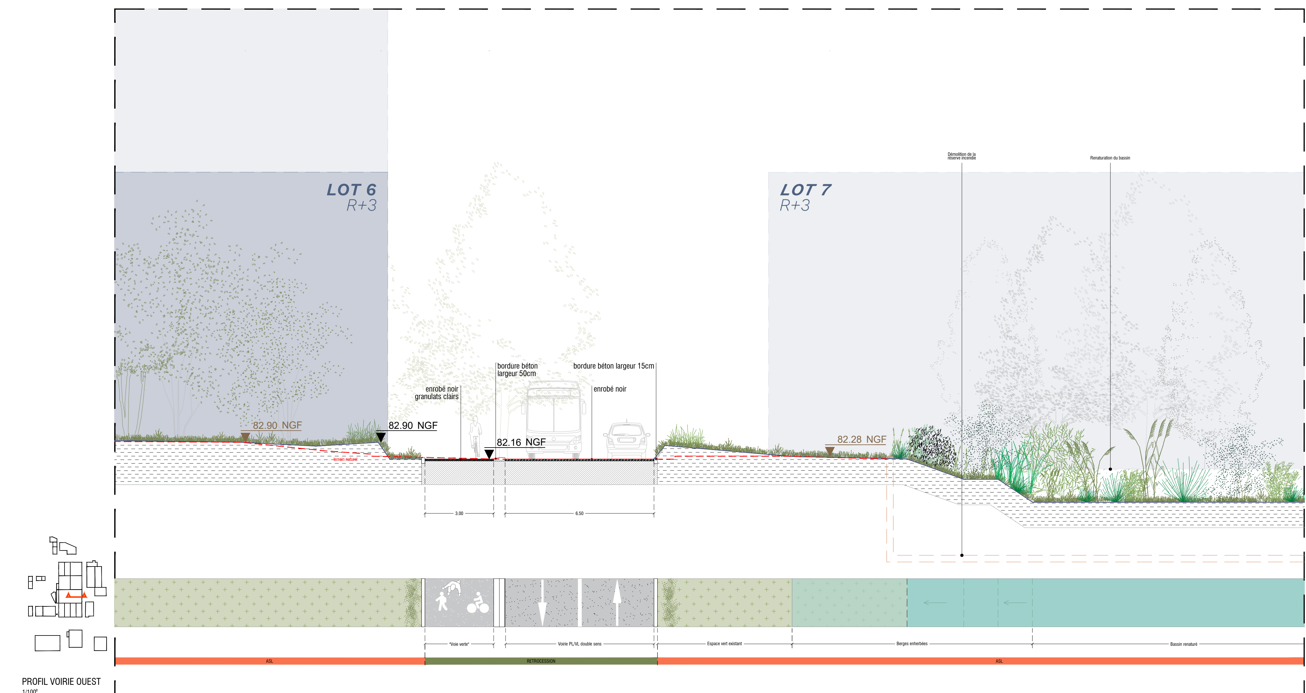
PROFIL VOIRIE OUEST 1/100'
