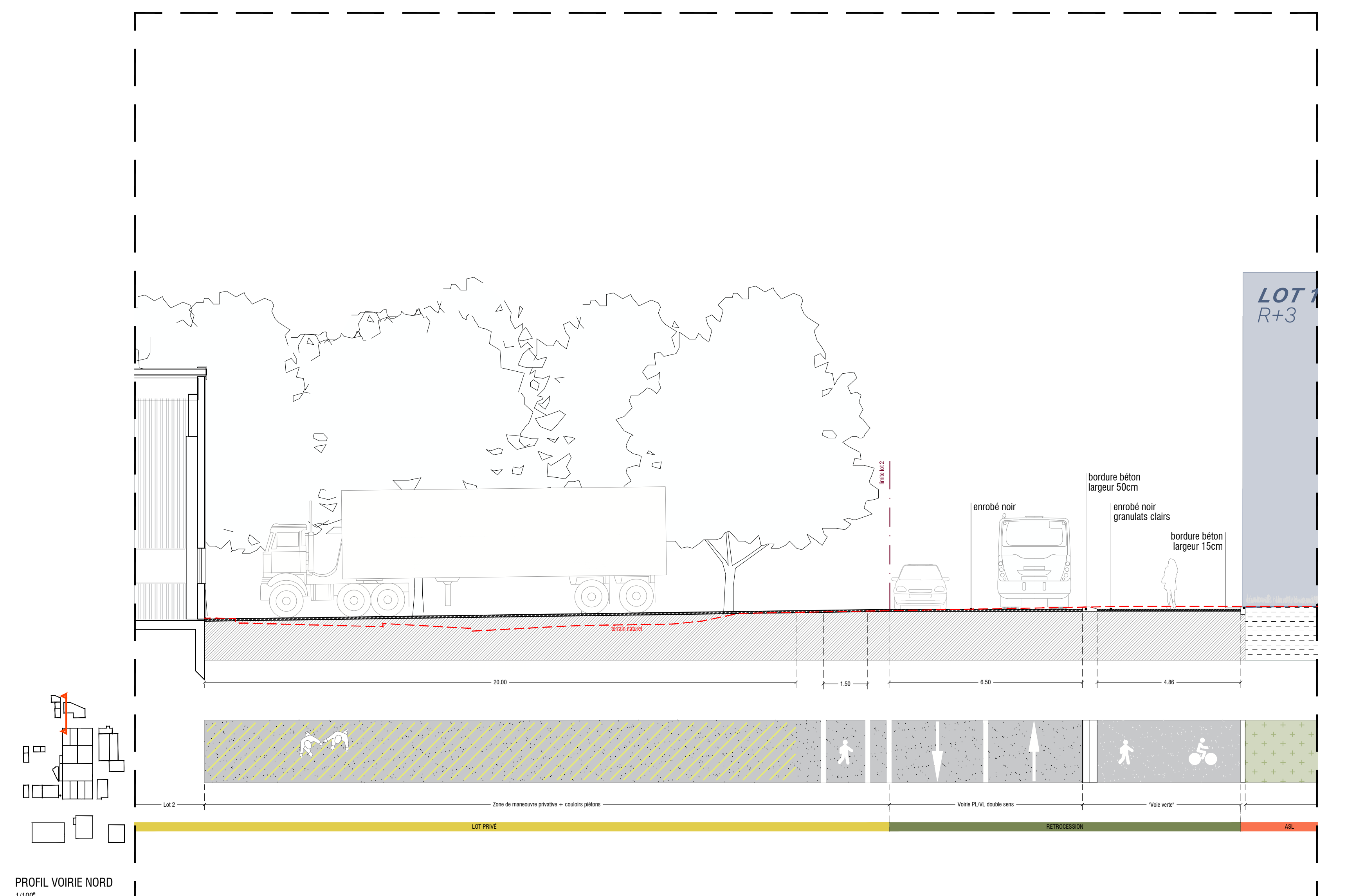
PROFIL VOIRIE NORD 1/100'
