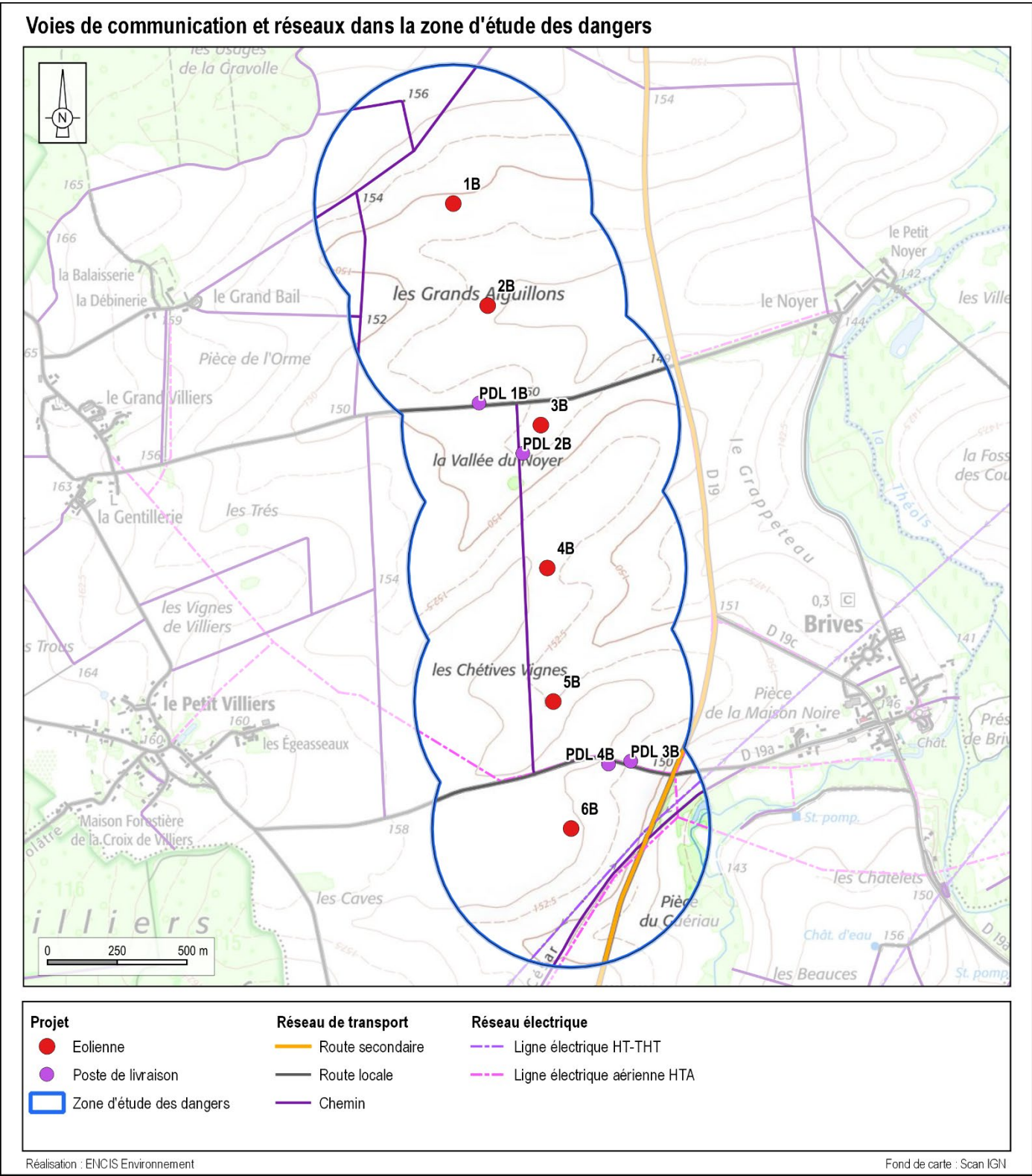
Carte 11 : Les infrastructures de transport identifiées au sein de la zone d'étude des dangers
