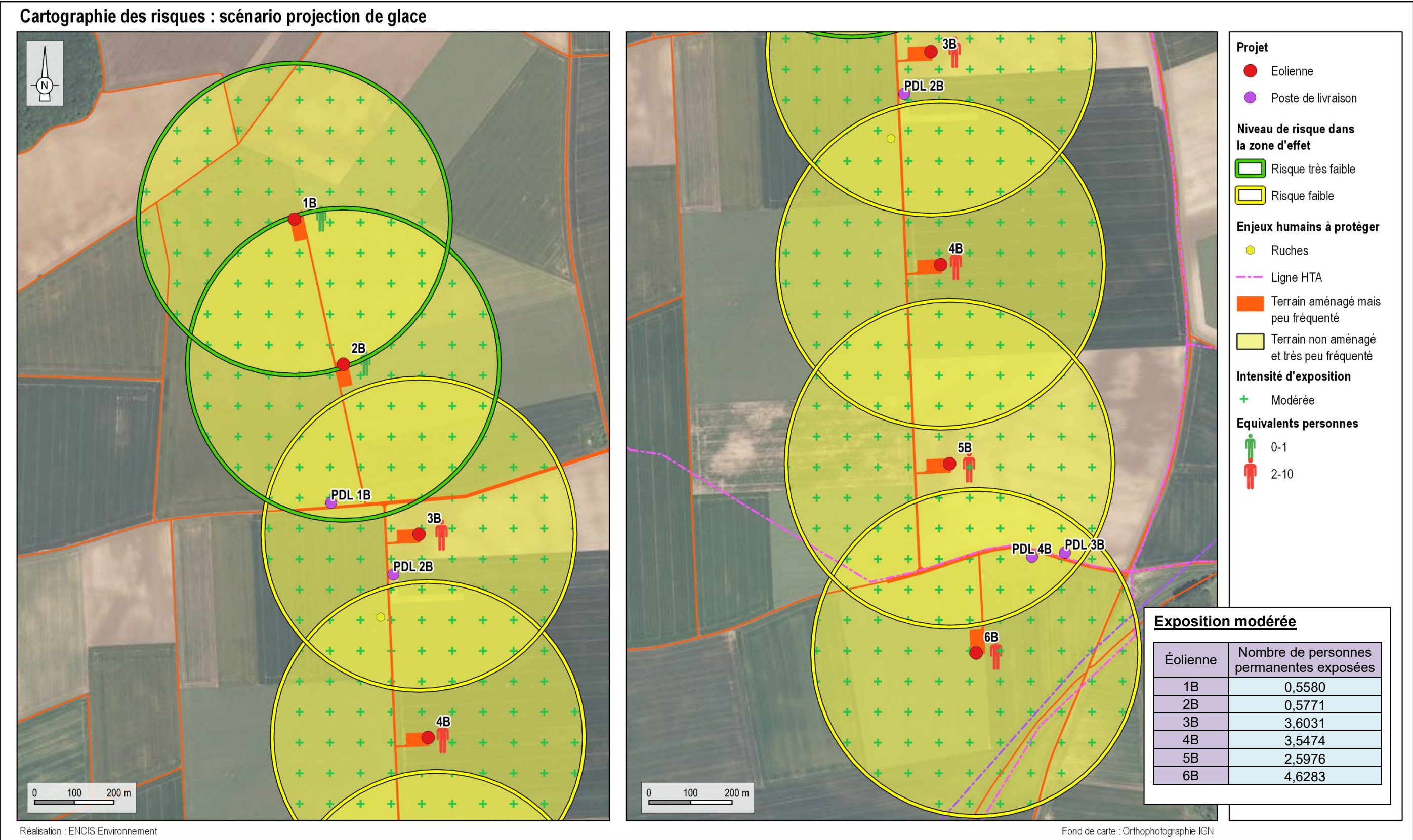
Carte 23 : Cartographie des risques – Scénario de projection de morceaux de glace
