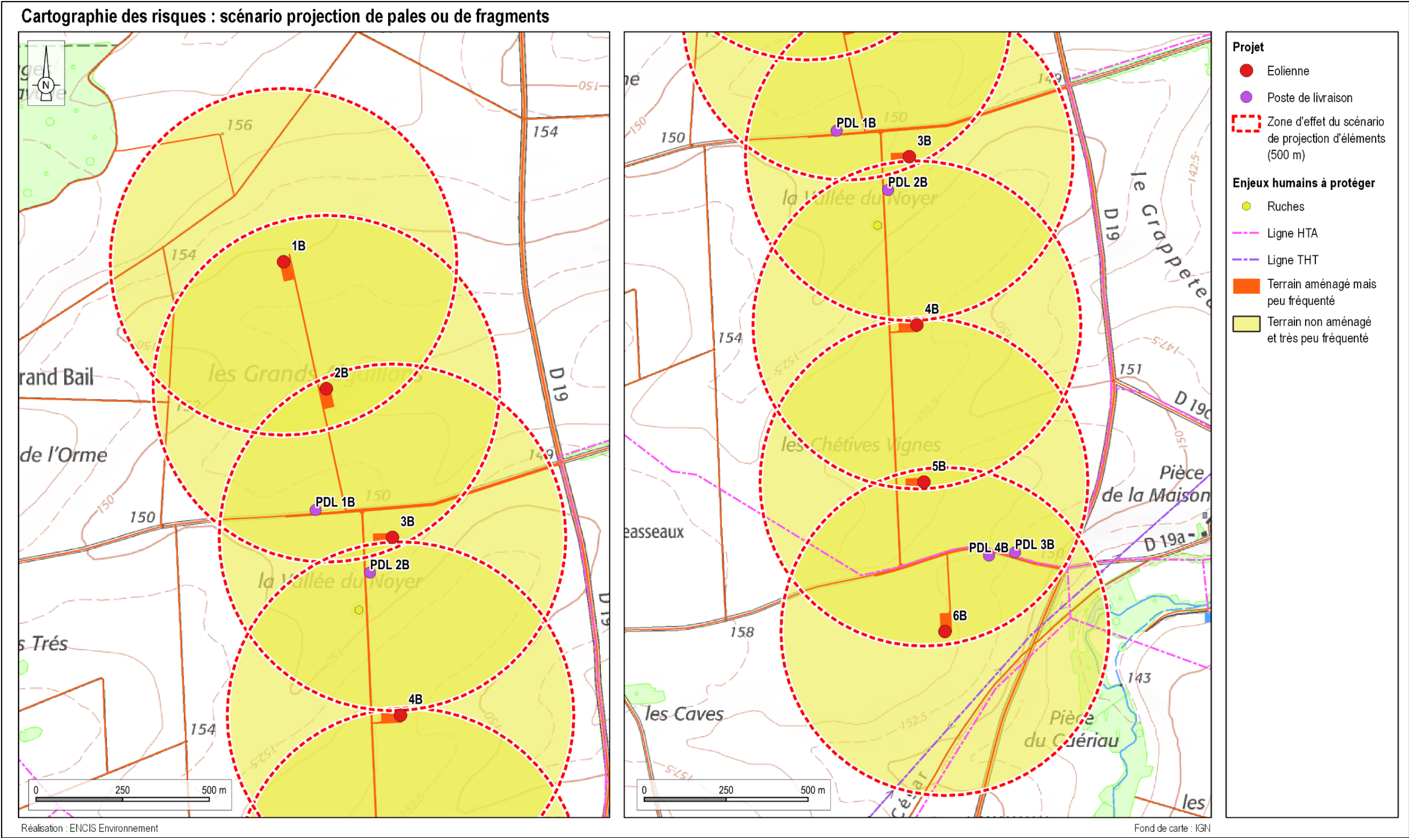
Carte 17 : Cartographie des enjeux identifiés dans les zones d'effet du scénario de projection de pales ou de fragments de pales
