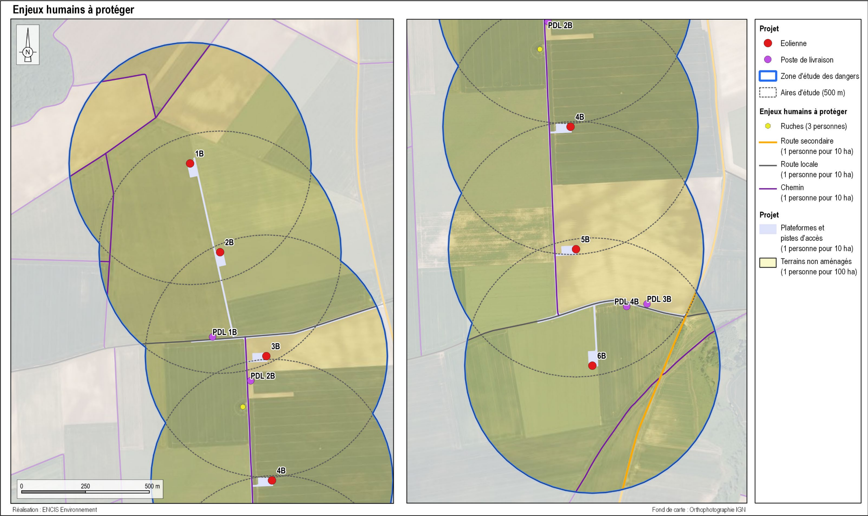
Carte 12 : Les intérêts à protéger (enjeux) au sein des aires d'étude des dangers des éoliennes des Grands Aiguillons 2
