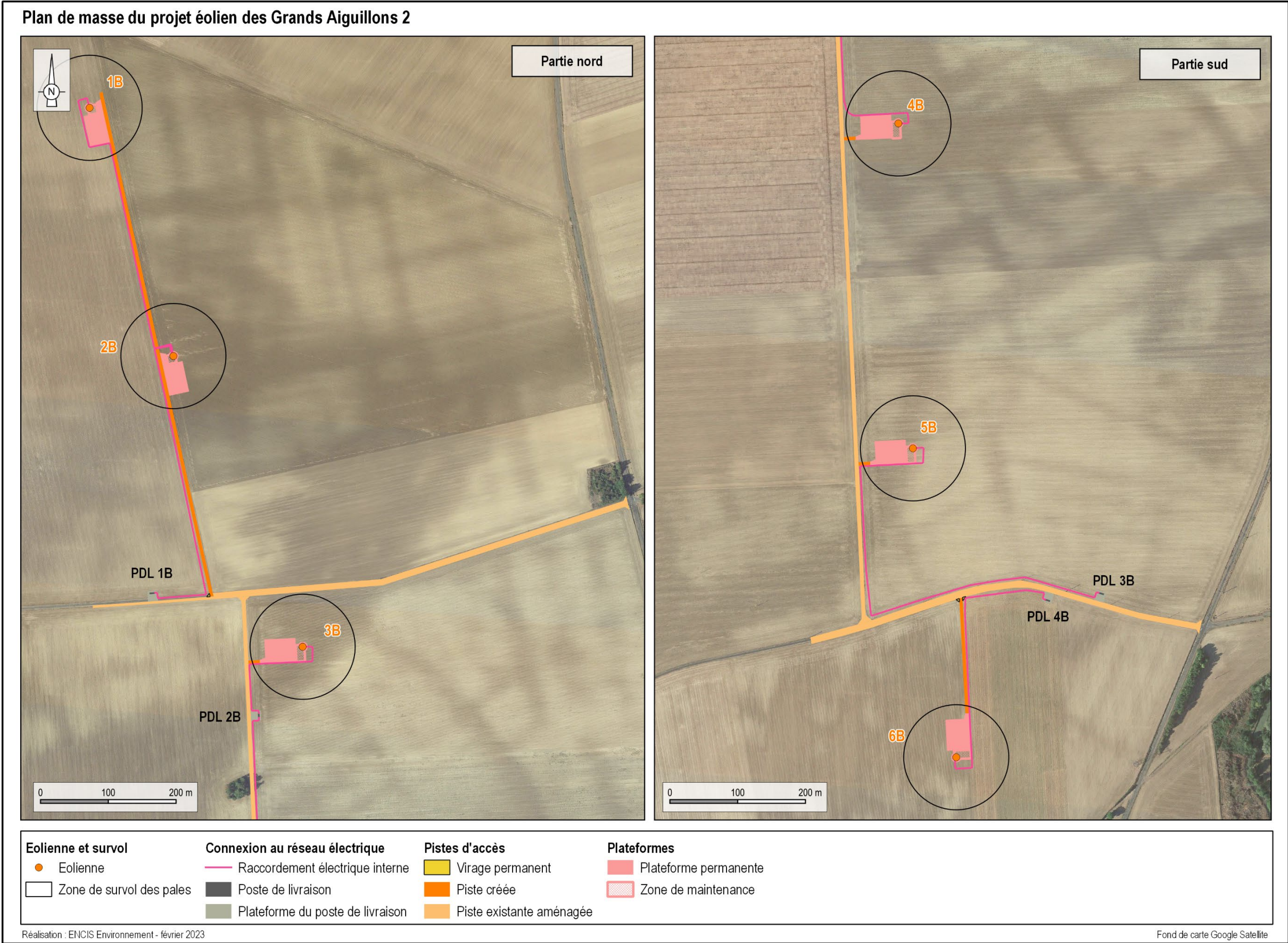
Carte 6 : Plan du projet de parc éolien des Grands Aiguillons 2
