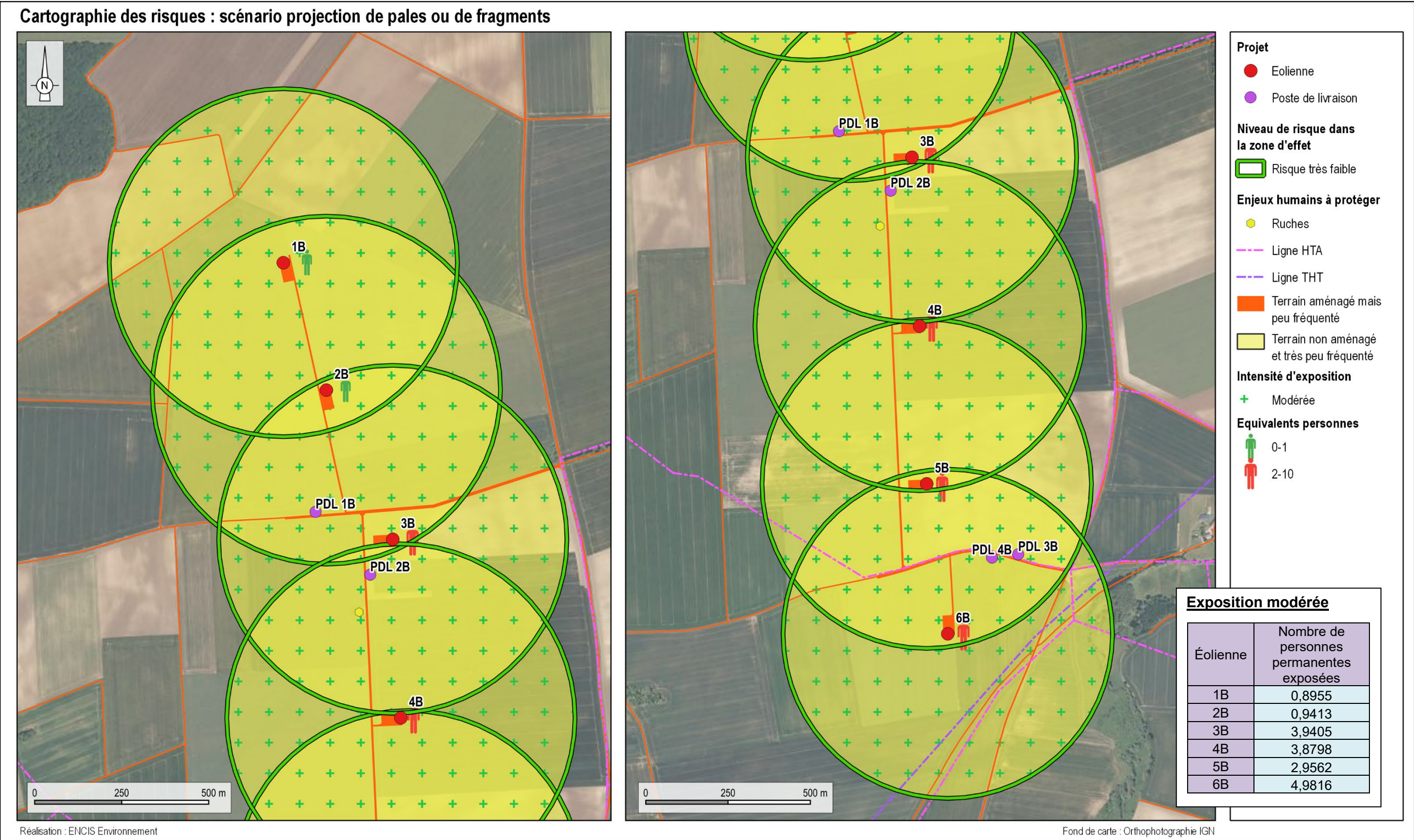
Carte 10 : Cartographie des risques – Scénario de projection de pales ou de fragments de pales
