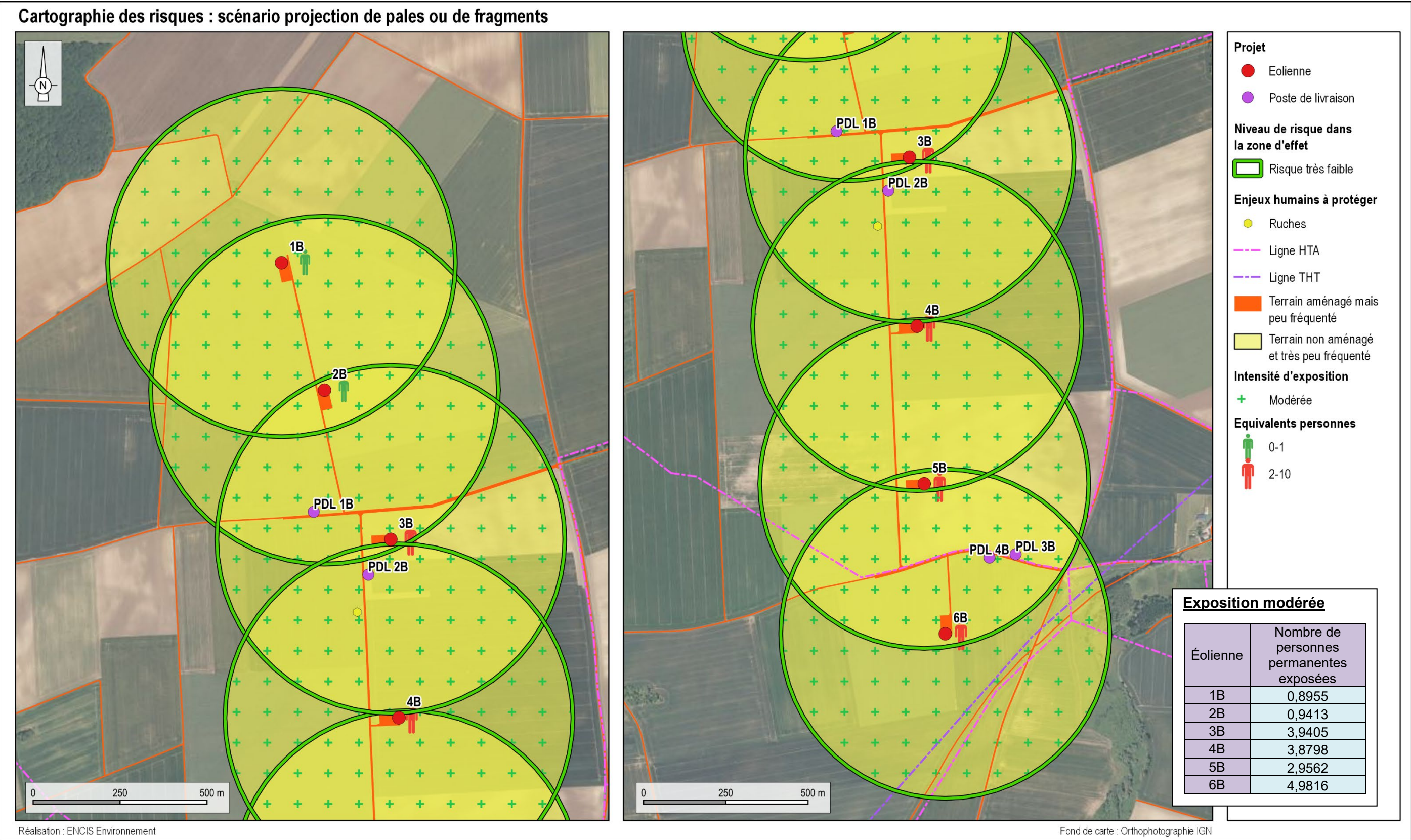
Carte 22 : Cartographie des risques – Scénario de projection de pales ou de fragments de pales
