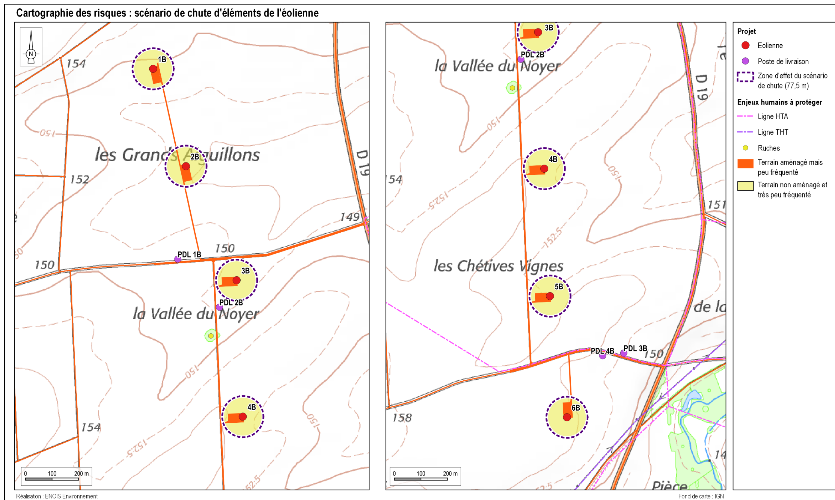
Carte 16 : Cartographie des enjeux identifiés dans les zones d'effet du scénario de chute d'éléments
