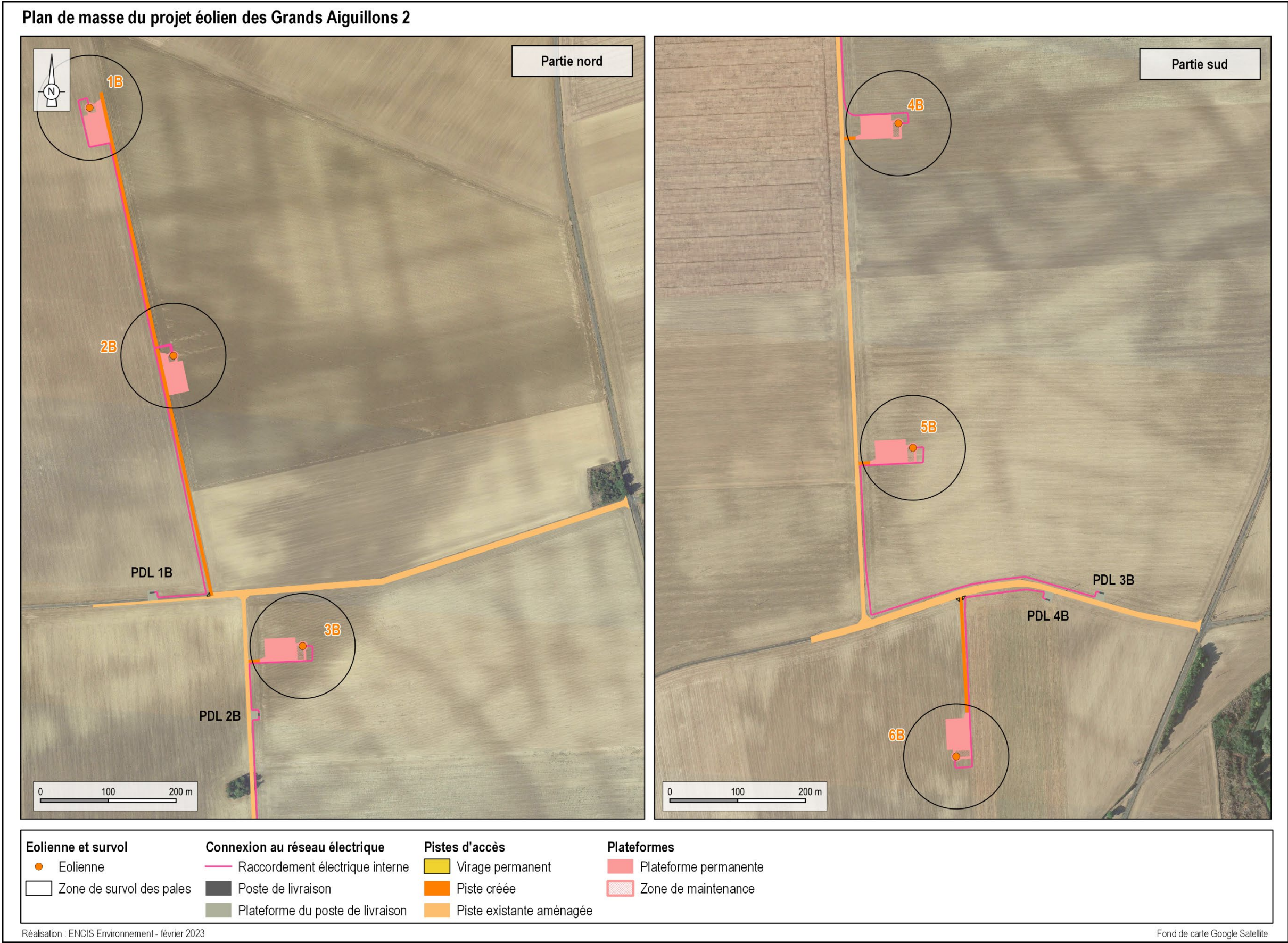
Carte 13 : Plan du projet de parc éolien des Grands Aiguillons 2
