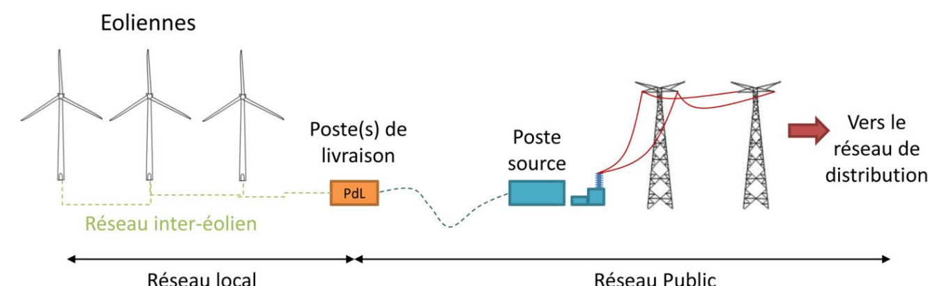
Figure 5 : Raccordement électrique des installations (Source : Guide technique, mai 2012)
