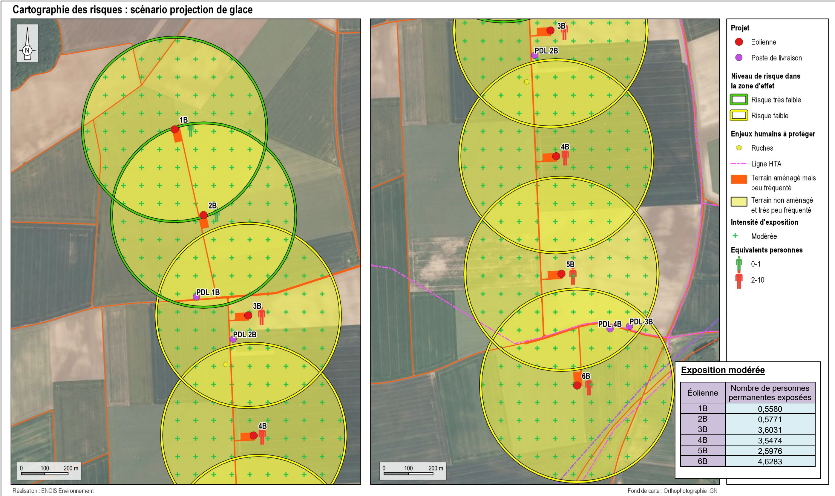
Carte 11 : Cartographie des risques – Scénario de projection de morceaux de glace
