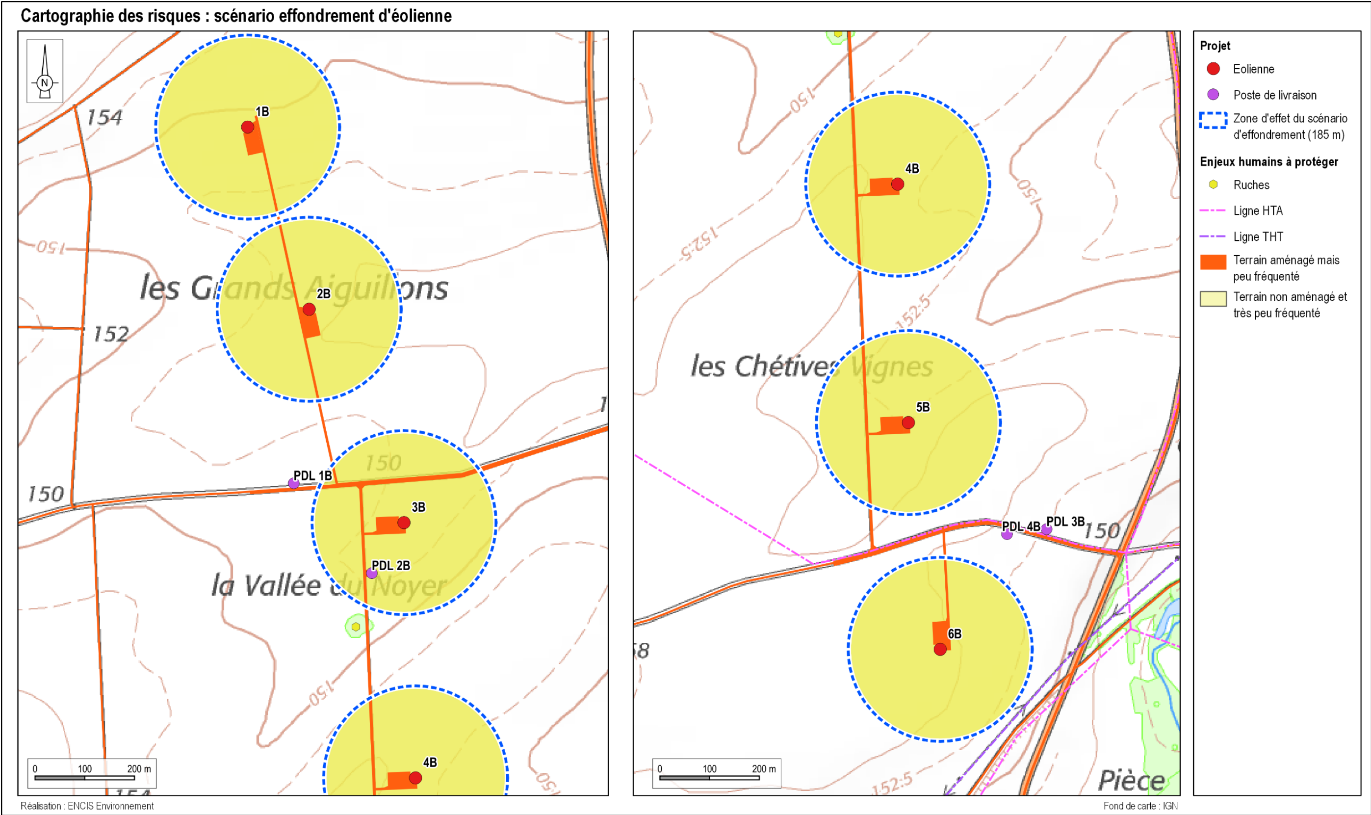
Carte 14 : Cartographie des enjeux identifiés dans les zones d'effet du scénario d'effondrement d'éolienne
