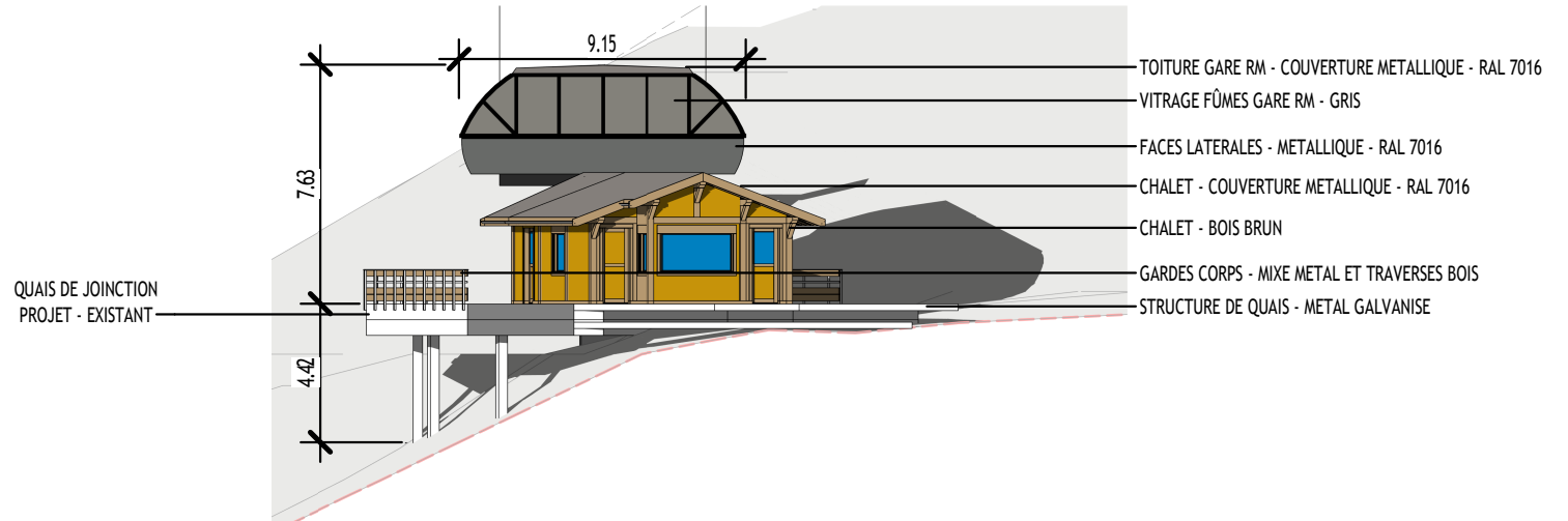
EST - AVAL - PIGNON CHALET 1 : 250
