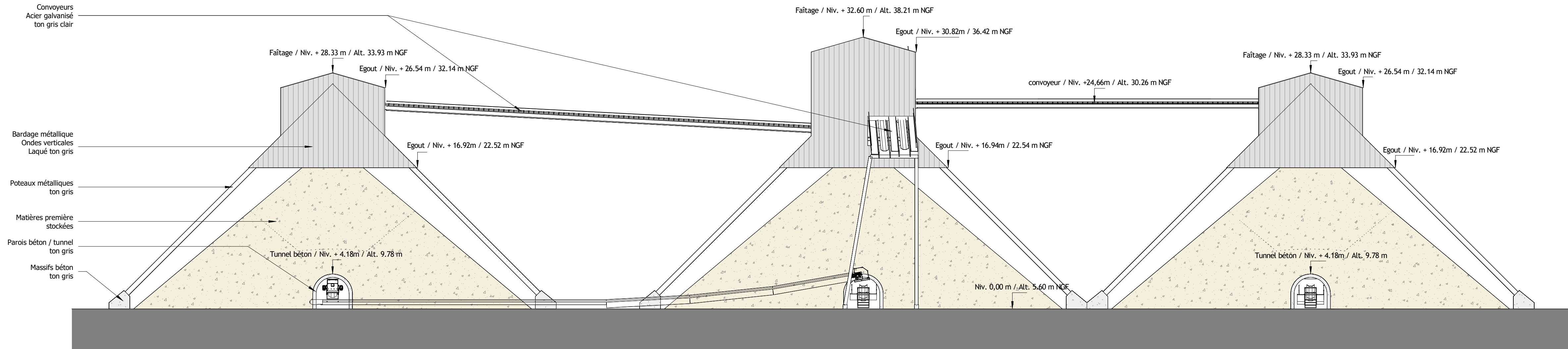
Façade OUEST / Ech. 1-300
