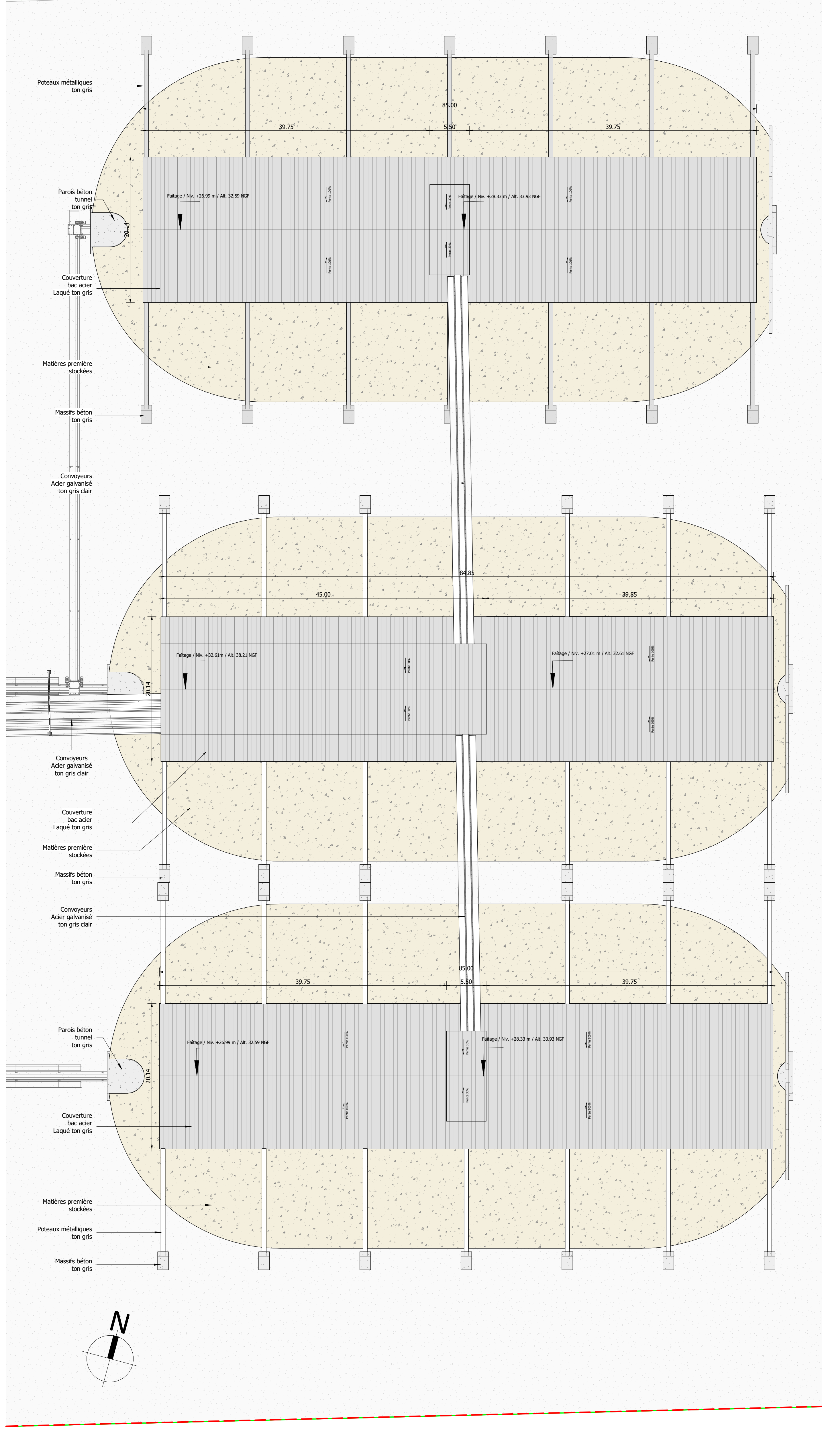
PLAN DE TOITURE / Ech. 1-300
