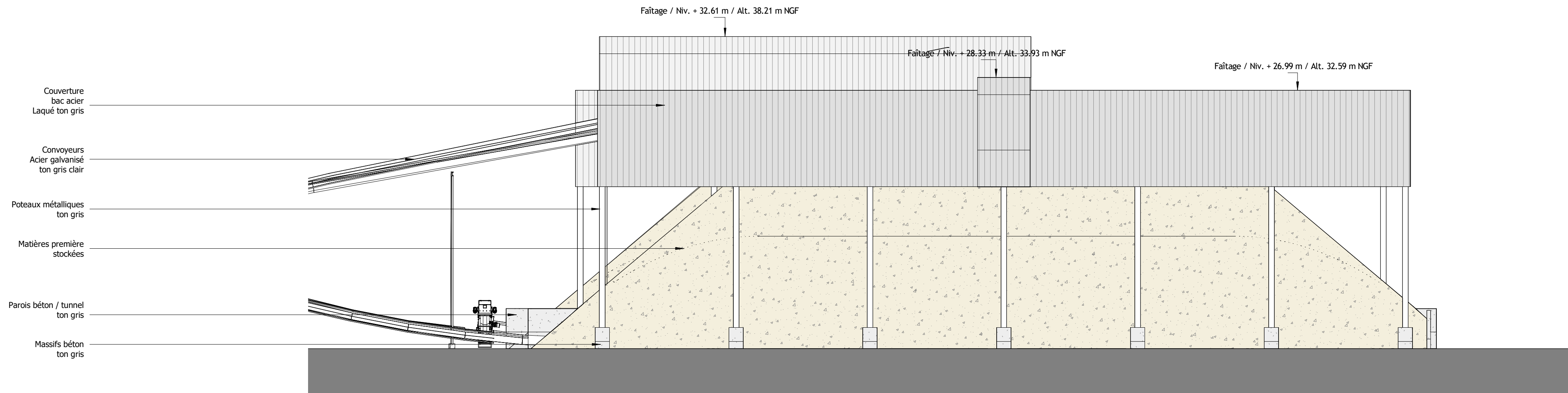
Façade SUD / Ech. 1-300
