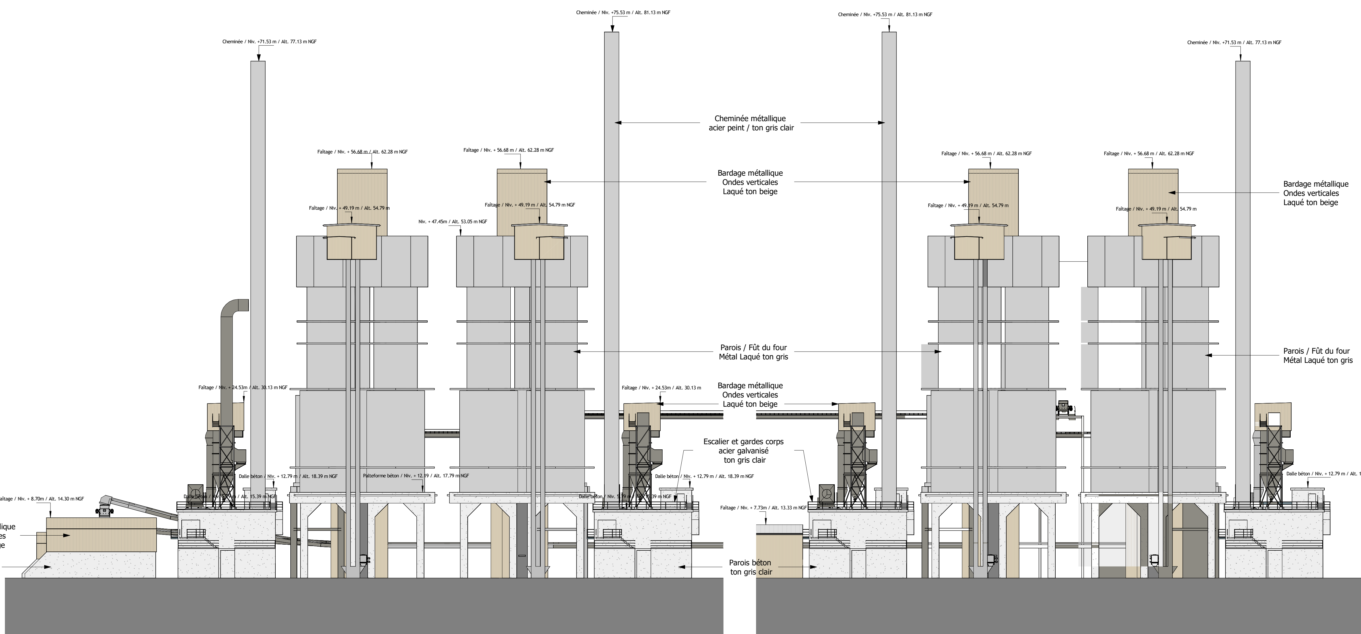
Repère 7 / Façade OUEST / Ech. 1-300
