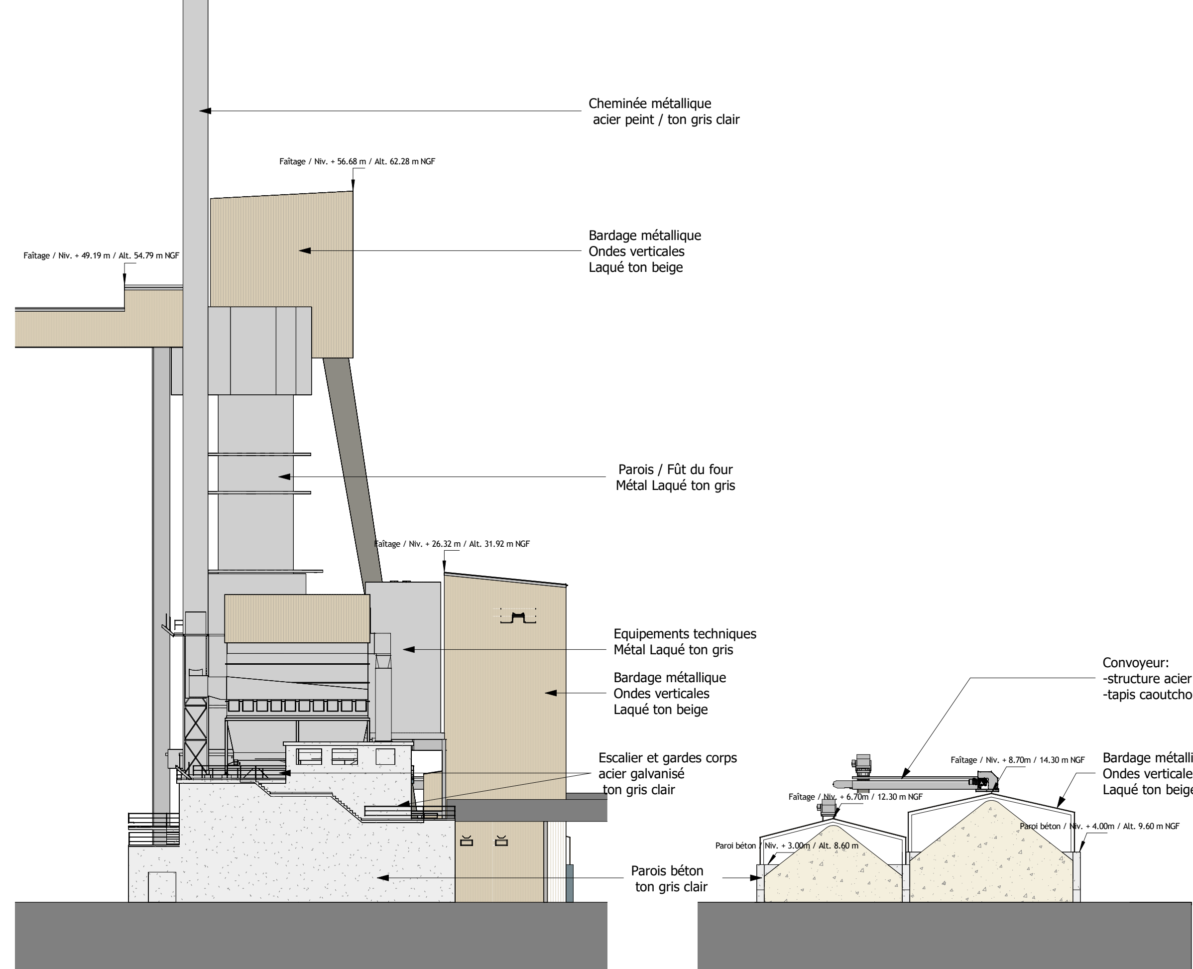
Repère 6 / Façade NORD / Ech. 1-300
