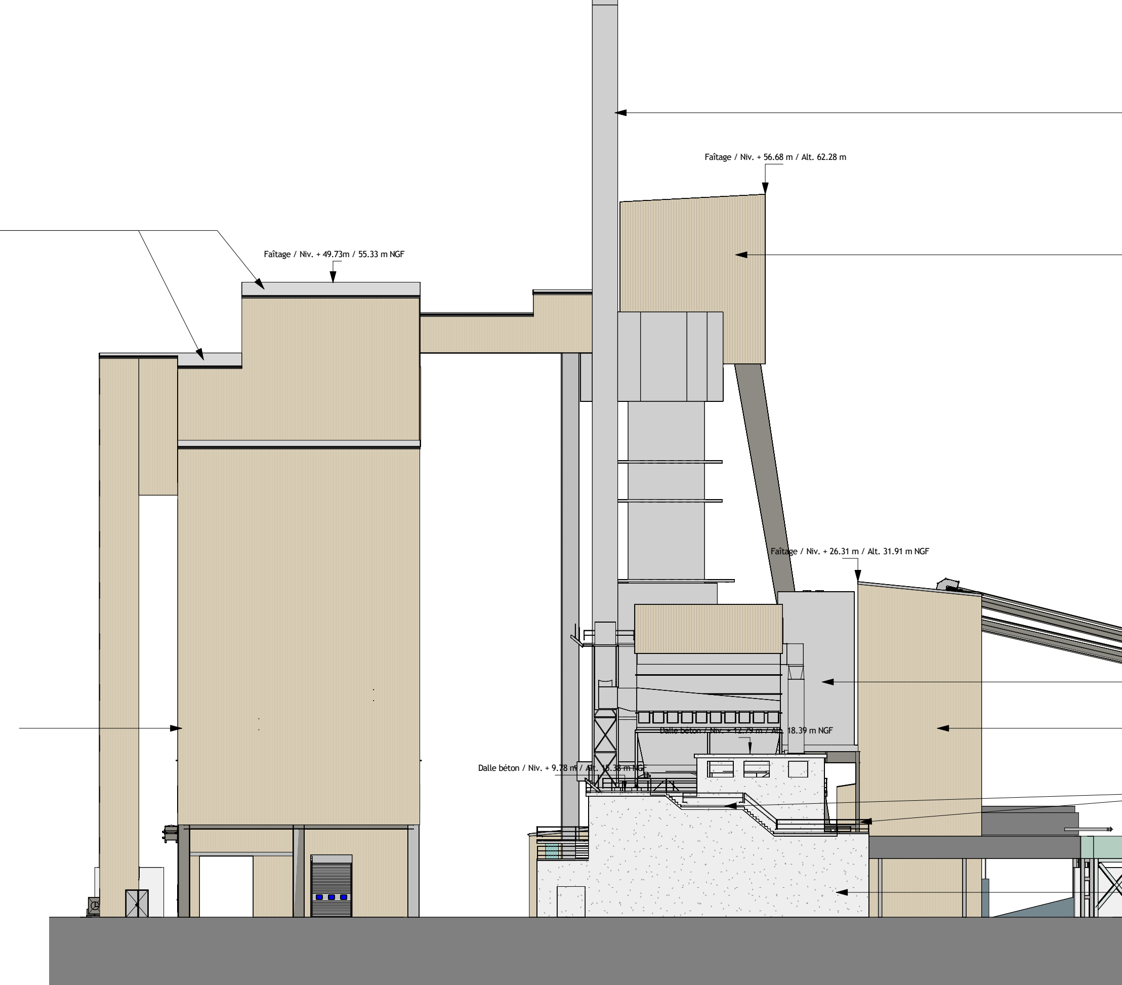
Repère 2 / Façade SUD / Ech. 1-300
