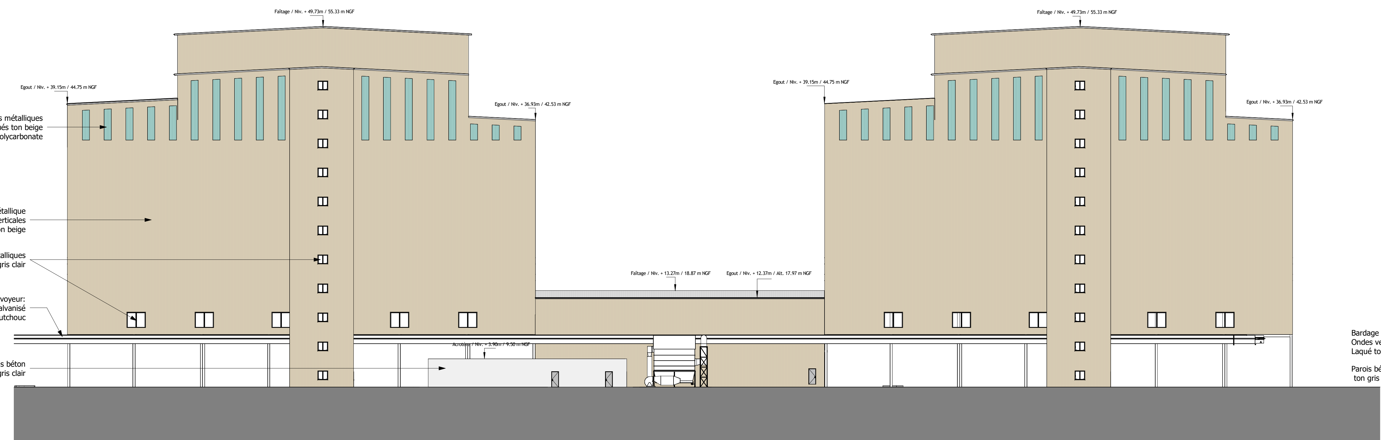
Repère 3 / Façade OUEST / Ech. 1-300
