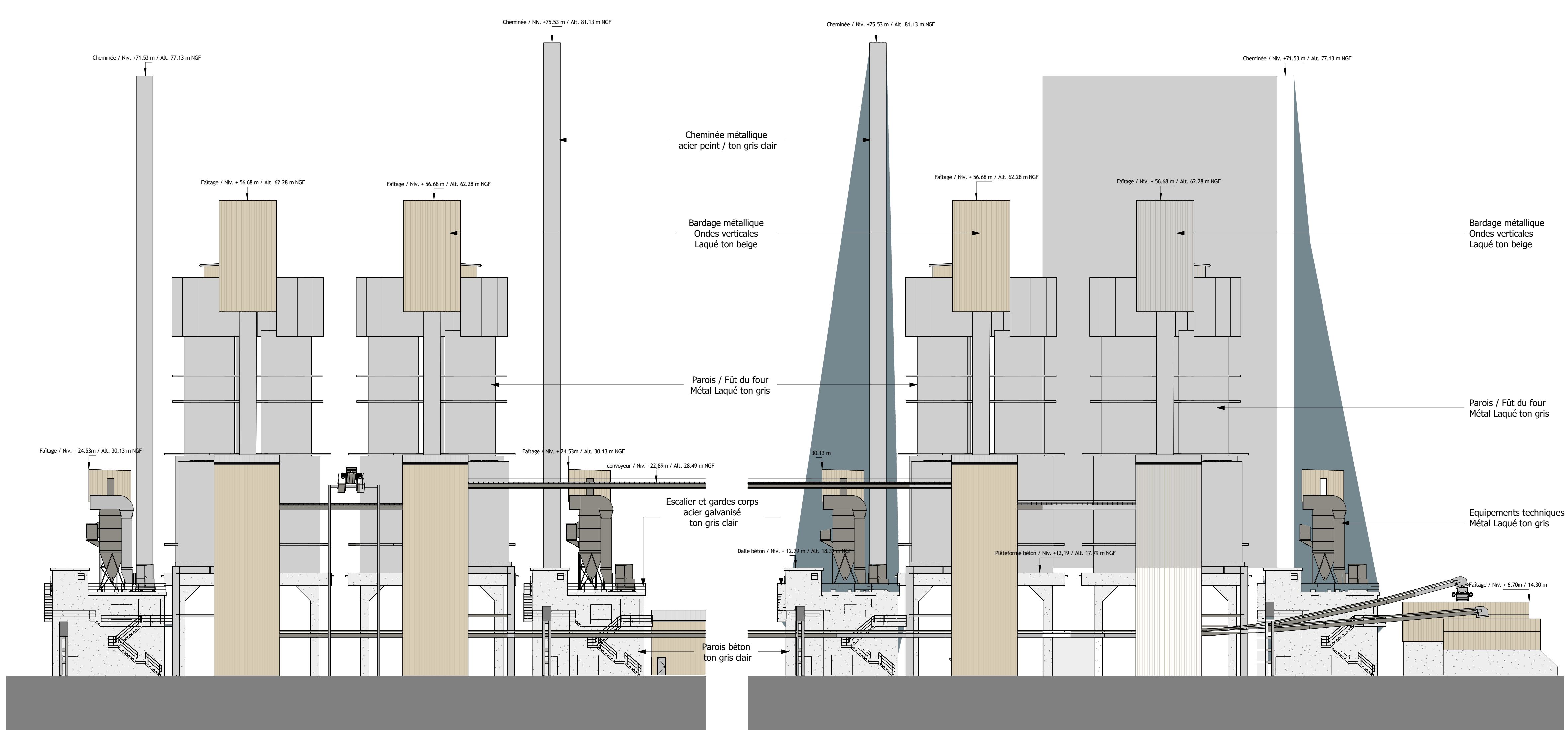
Repère 9 / Façade EST / Ech. 1-300
