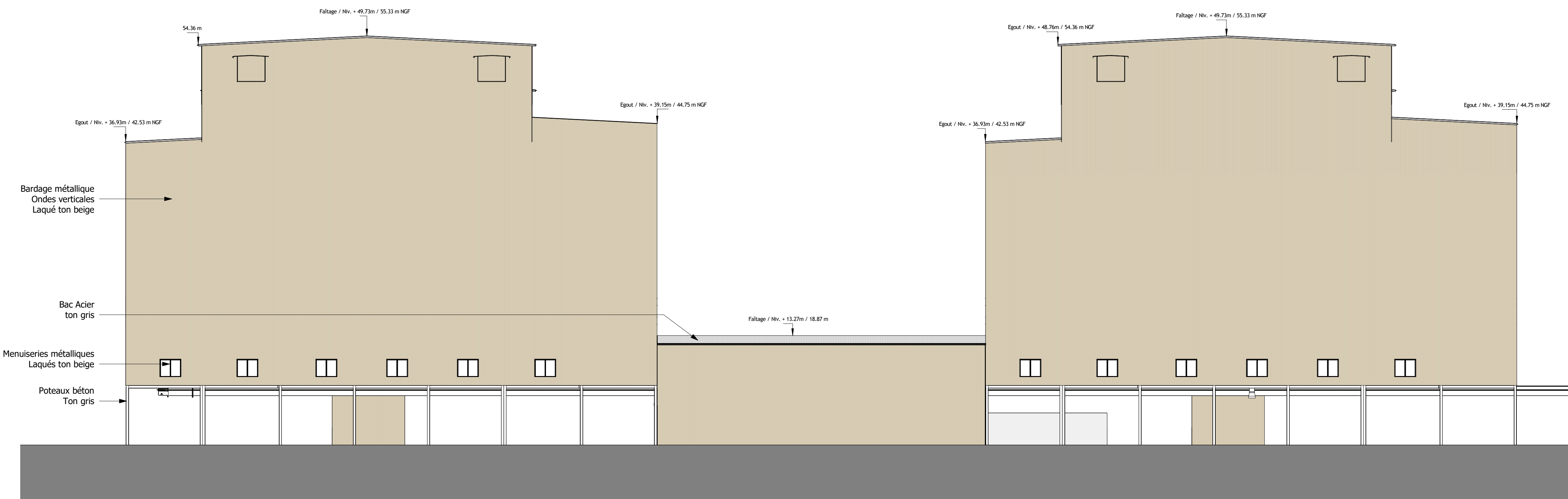
Repère 4 / Façade EST / Ech. 1-300
