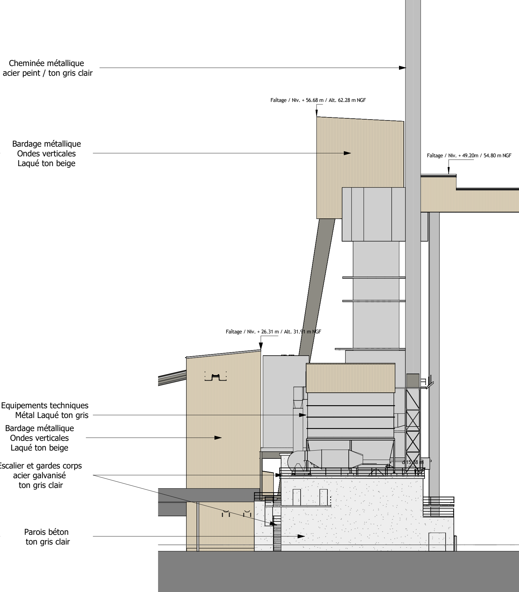
Repère 5 / Façade SUD / Ech. 1-300
