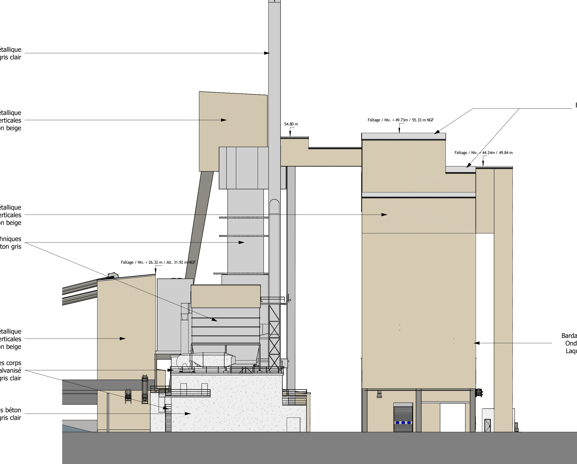
Repère 1 / Façade NORD / Ech. 1-300
