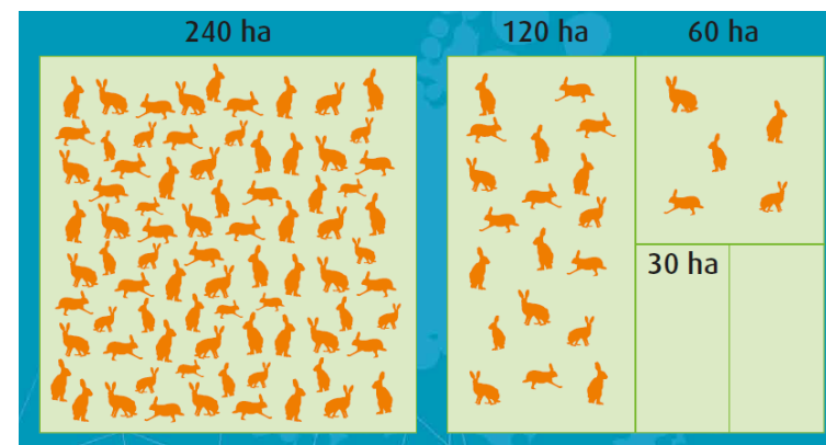
Figure 18 : Effet de la fragmentation du territoire sur les populations : cas du Lièvre commun sur le plateau suisse
