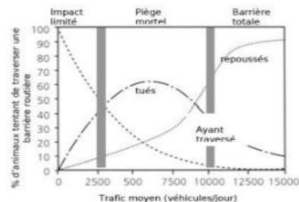
Figure 1: Effet de fragmentation des infrastructures routières en fonction du trafic moyen journalier (Source : IUELL et al. 2007).
