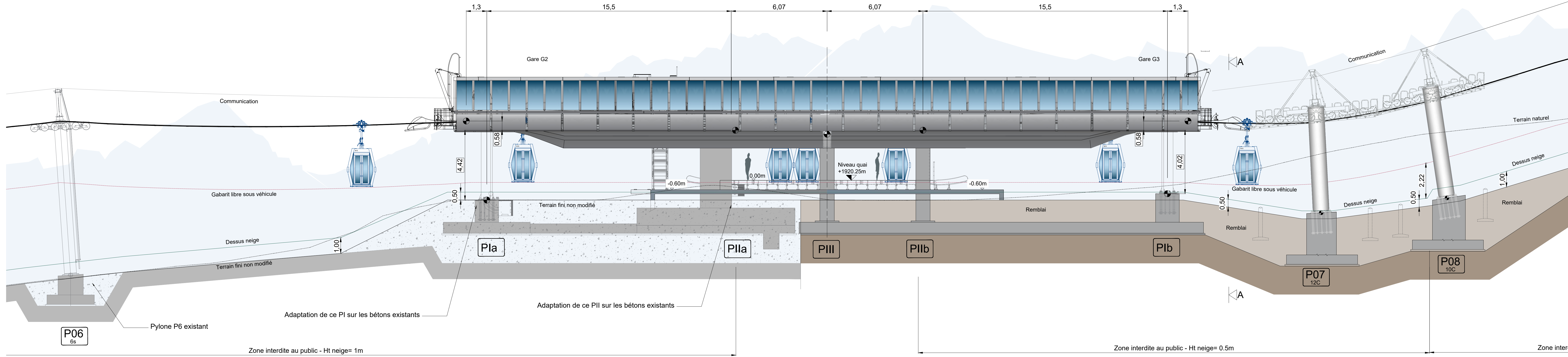
G2 Vue longitudinale BB
