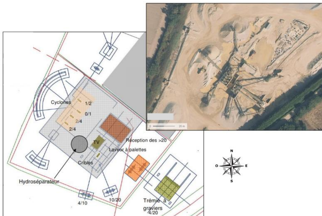
Plan des installations de traitement
