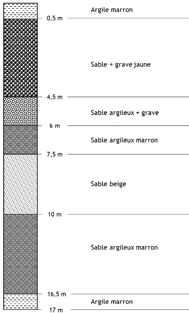
Figure 14. Coupe du gisement du sondage A47 sur la zone de l'extension Source : HMFG
