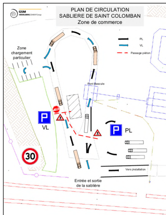
Figure 23. Plan de circulation actuel sur la plateforme de commercialisation Source : HMFG
