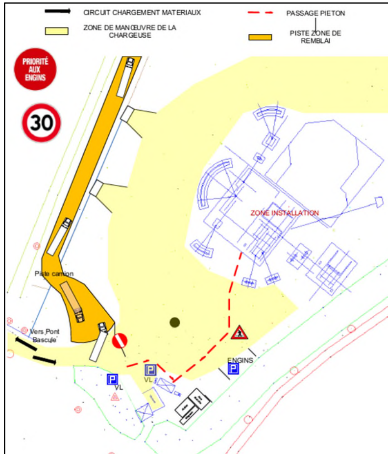
Figure 24. Plan de circulation actuel au niveau des installations de traitement des matériaux Source : HMFG
