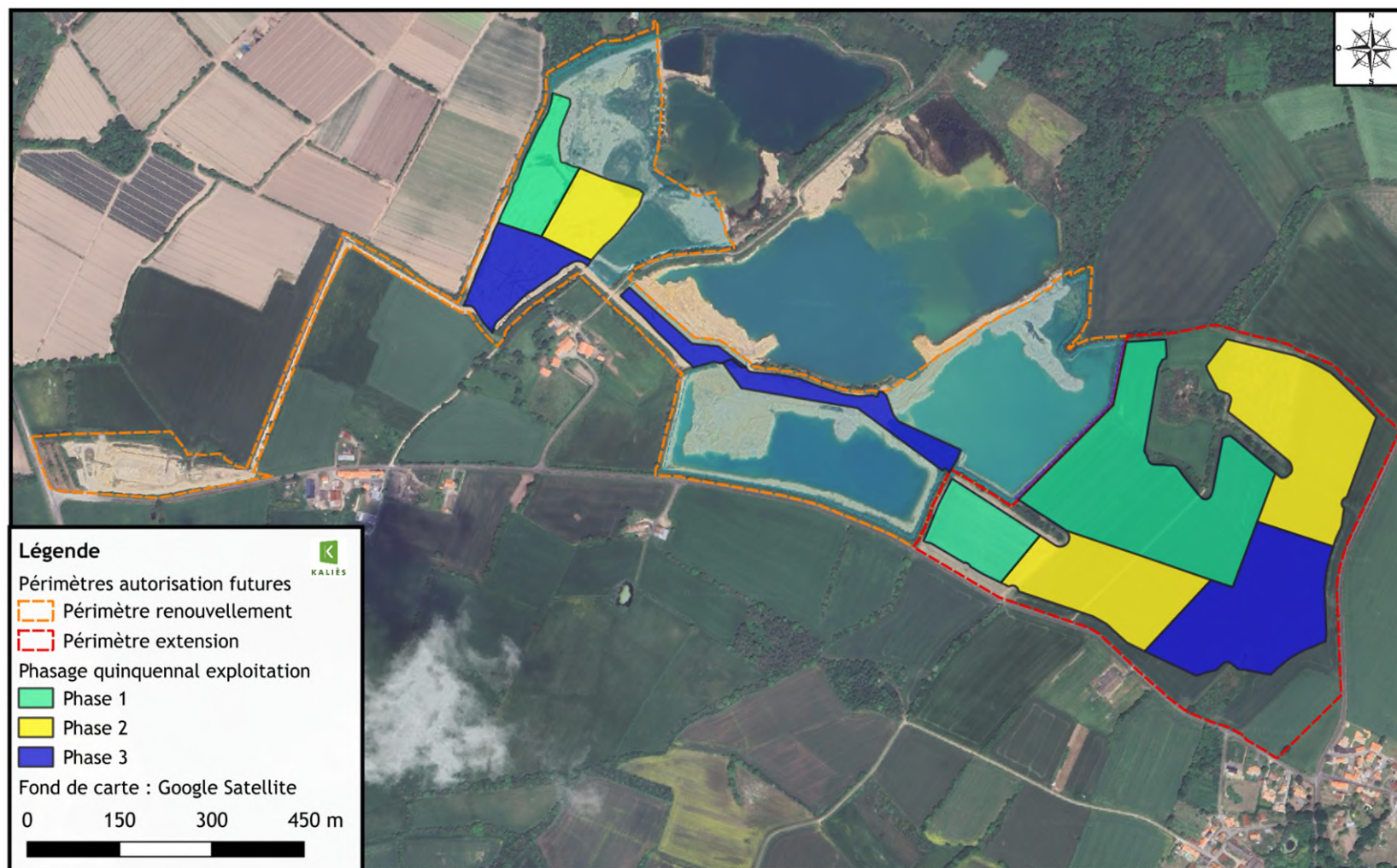
Figure 34. Phasage de l'exploitation de l'extension de la carrière Source : HMFG
