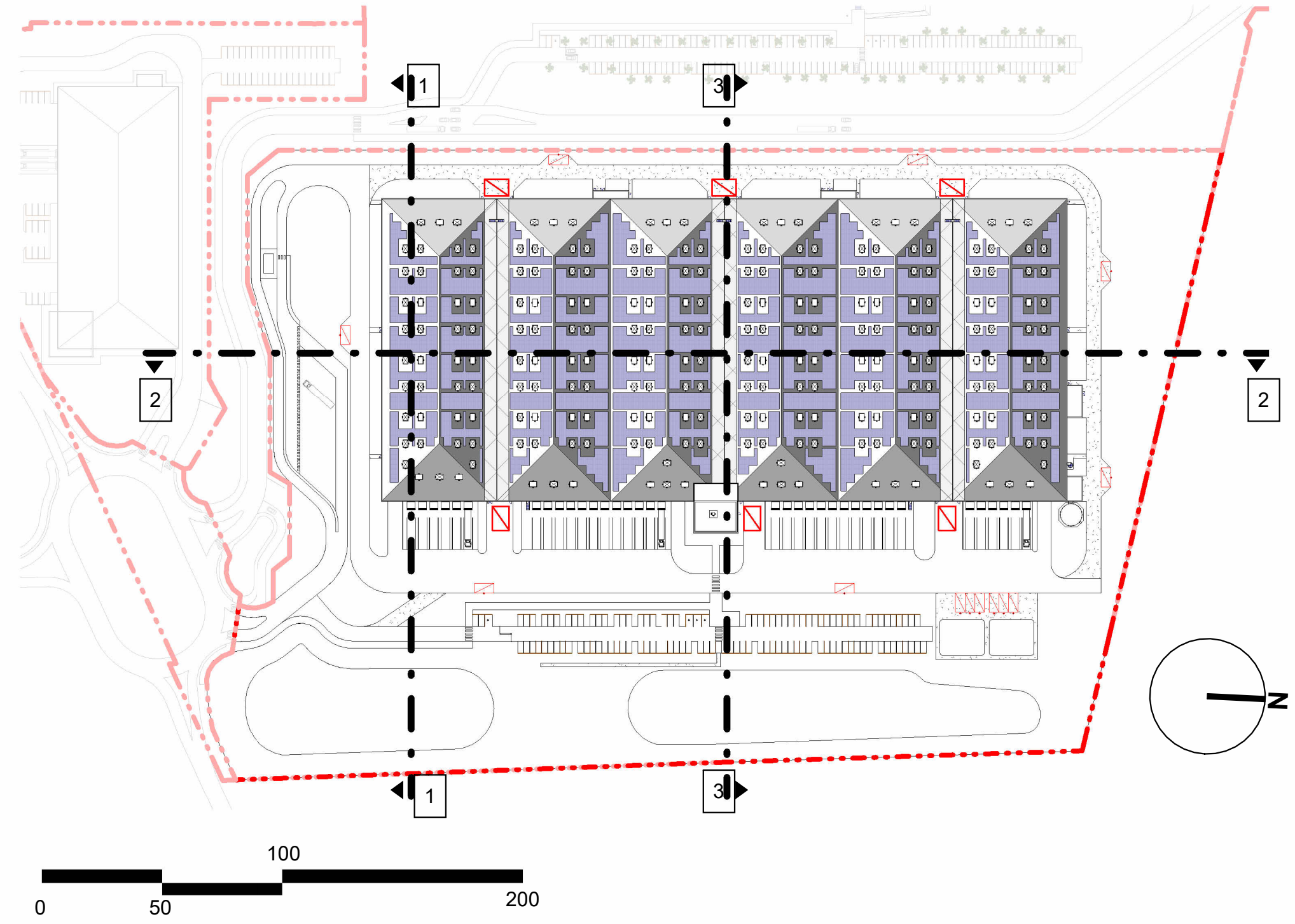
4 PLAN DE REPERAGE DES COUPES 1 : 2000
