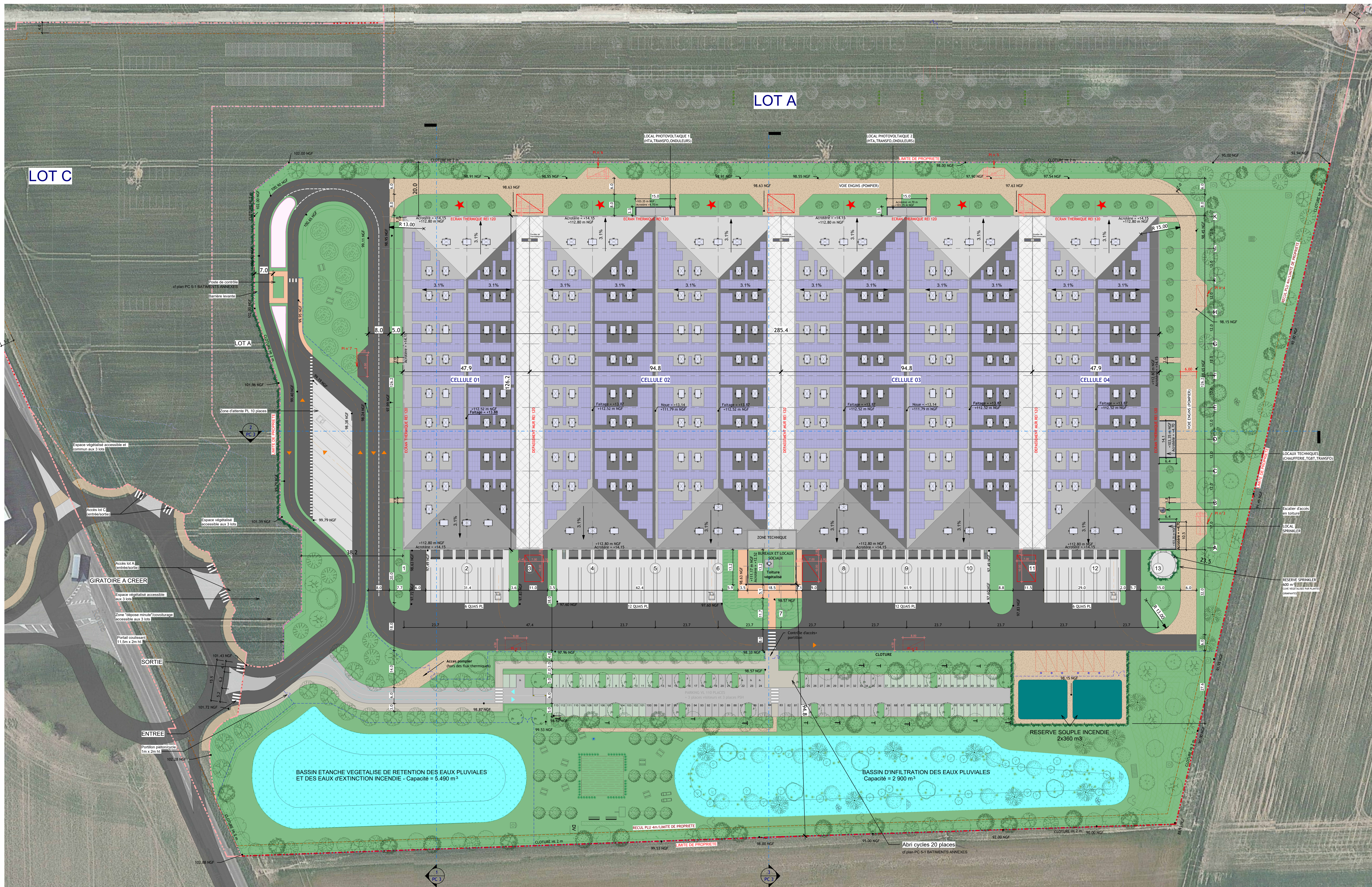
1 PLAN MASSE 1 : 500
