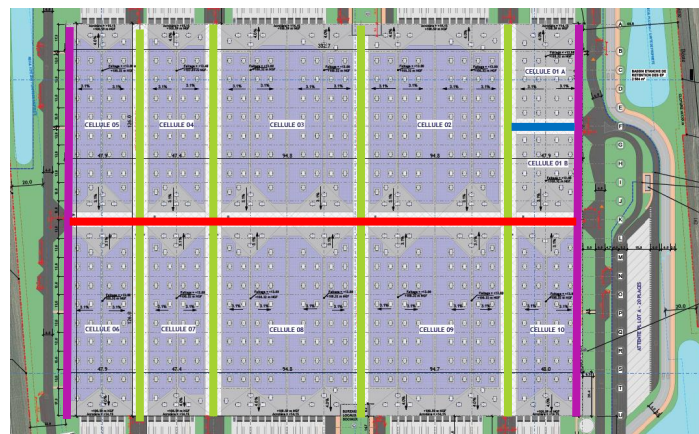
Figure 30 - Plan de compartimentage du bâtiment
