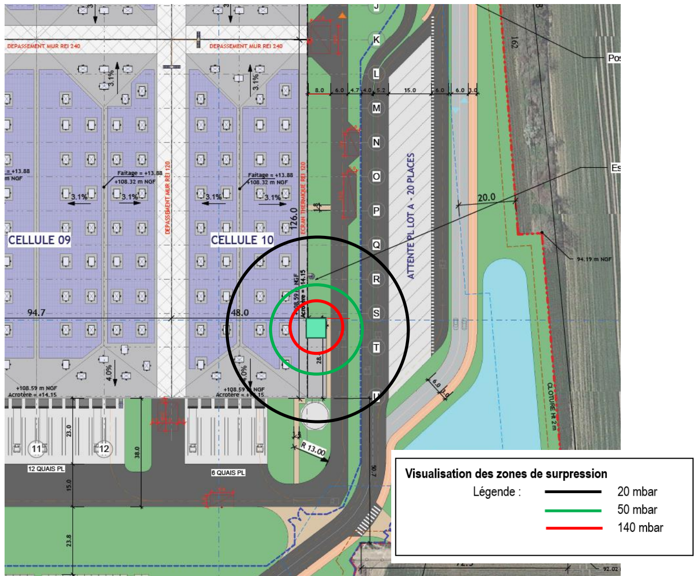
Carte des distances d'effets de suppression de la chaufferie
