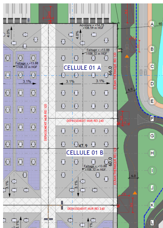
Figure 5 - Détail du découpage de la cellule 1
