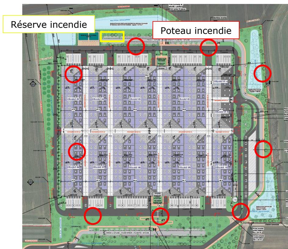
Figure 29 – Plan de l'organisation de la défense incendie sur le site
