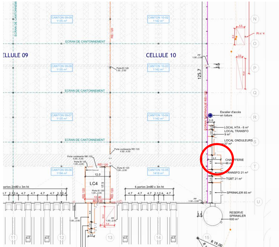
Figure 9 - Plan d'implantation de la chaufferie
