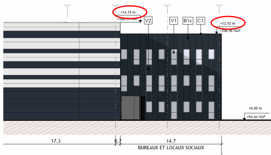
Figure 7 - Coupe de la façade Ouest du bâtiment
