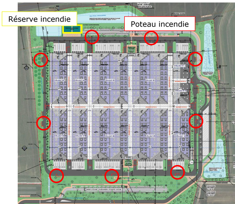
Figure 12 – Plan de l'organisation de la défense incendie sur le site
