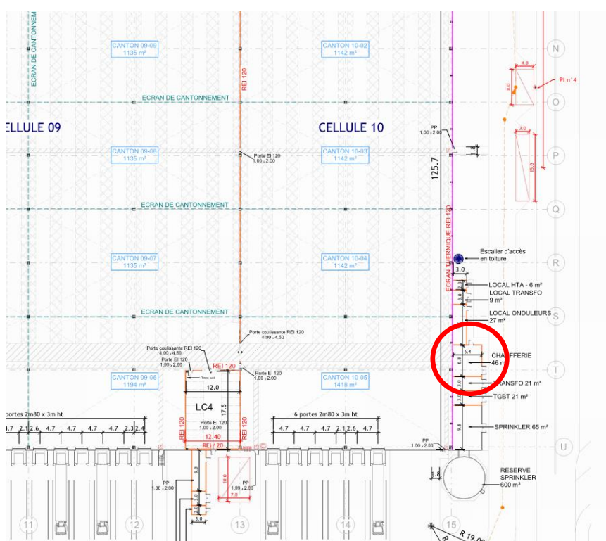
Figure 17 - Plan d'implantation de la chaufferie
