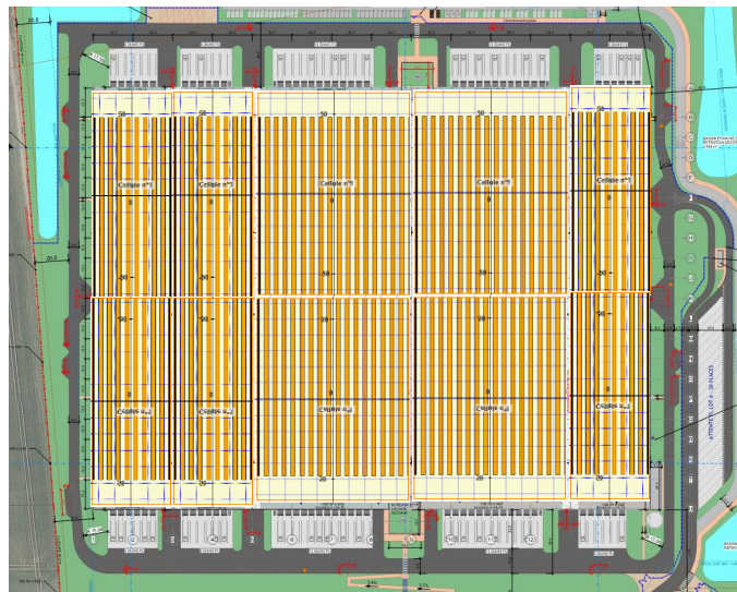
Figure 11 - Plan de rackage du bâtiment
