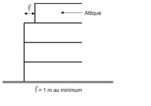
Schéma à titre illustratif
