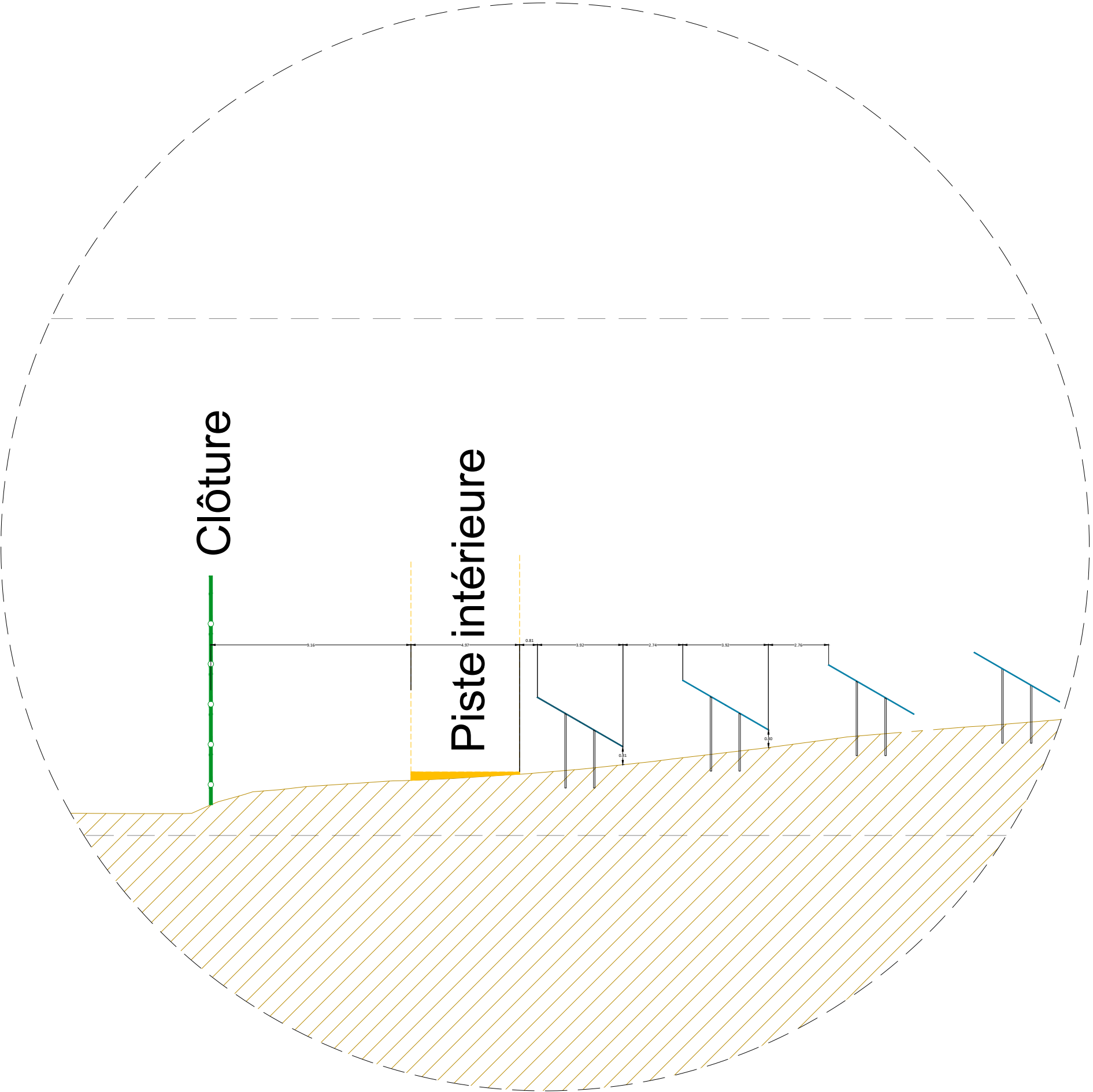
DÉTAIL 1 ÉCHELLE 1 / 200
