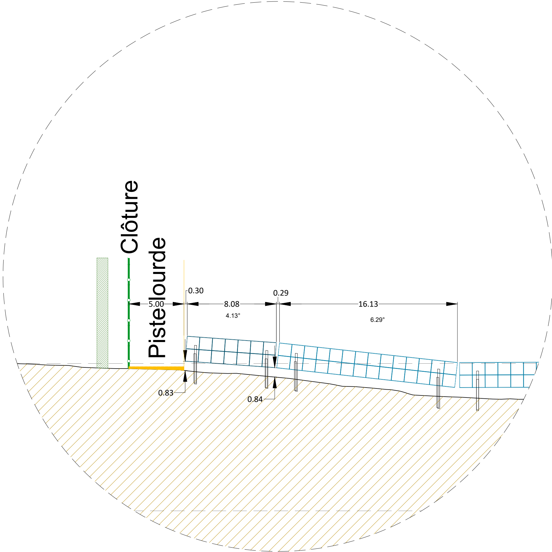
DÉTAIL 2 ÉCHELLE 1 / 200
