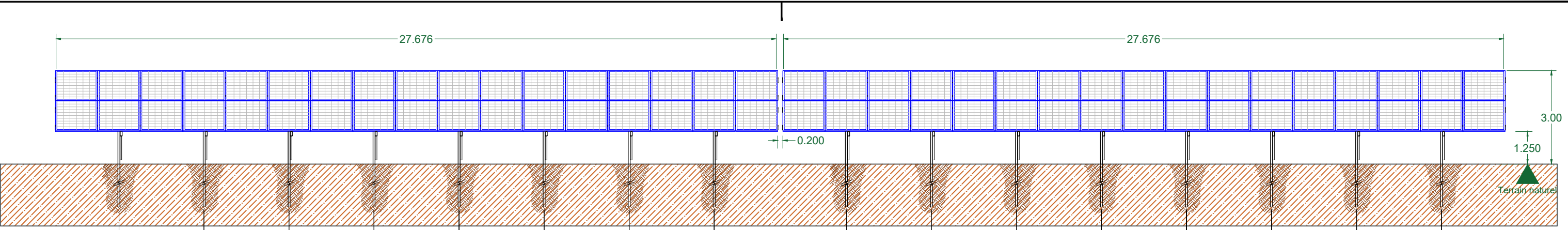
Vue de face d'une table:
