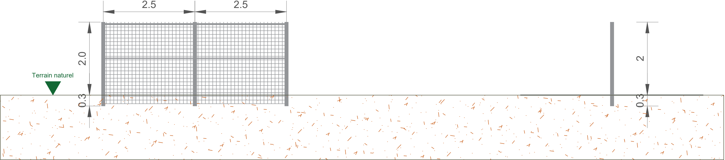
Vue de face de la clôture grillagée Maillage 15cm x 15cm
