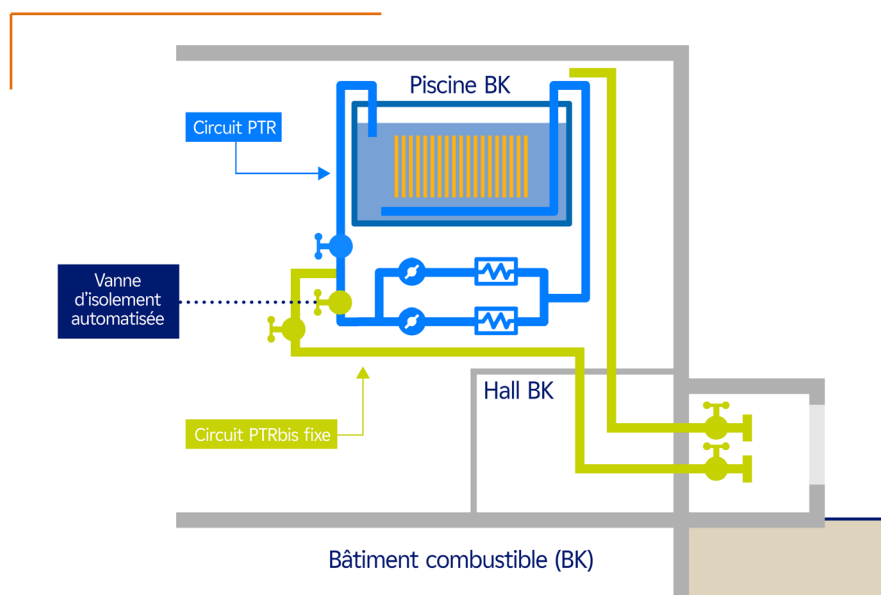
Figure 9. Disposition « Doublement du dispositif d'isolement automatique de la ligne d'aspiration de la piscine BK » : emplacement de la vanne
