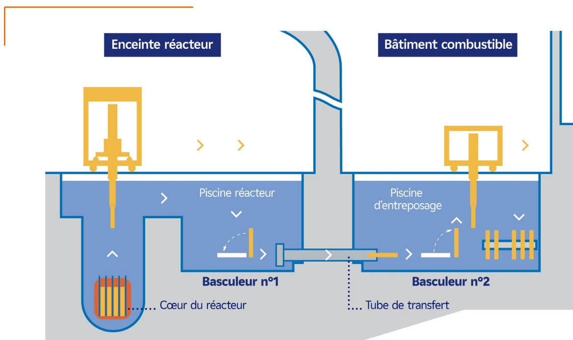
illustration 1. principe du transfert d'un assemblage de combustible du cœur du réacteur vers la piscine d'entreposage)
