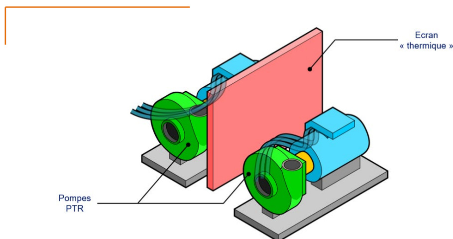
Figure 10. Installation d'un écran thermique entre les pompes du système de refroidissement de la piscine d'entreposage du combustible
