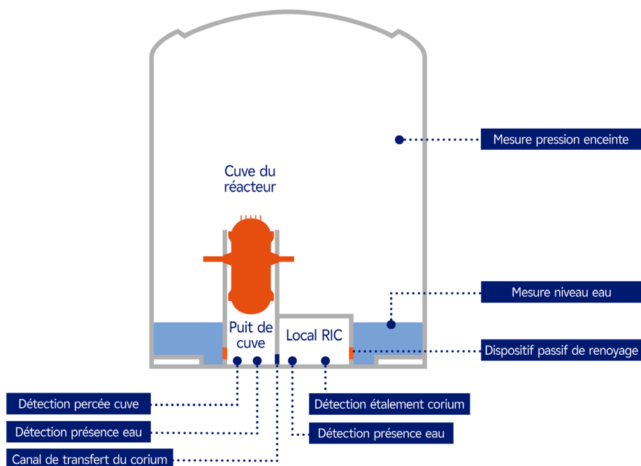
Figure 12. Illustration de la mesure de niveau d'eau dans les puisards du bâtiment réacteur et de la détection de l'étalement du corium dans le local d'instrumentation du cœur (RIC)
