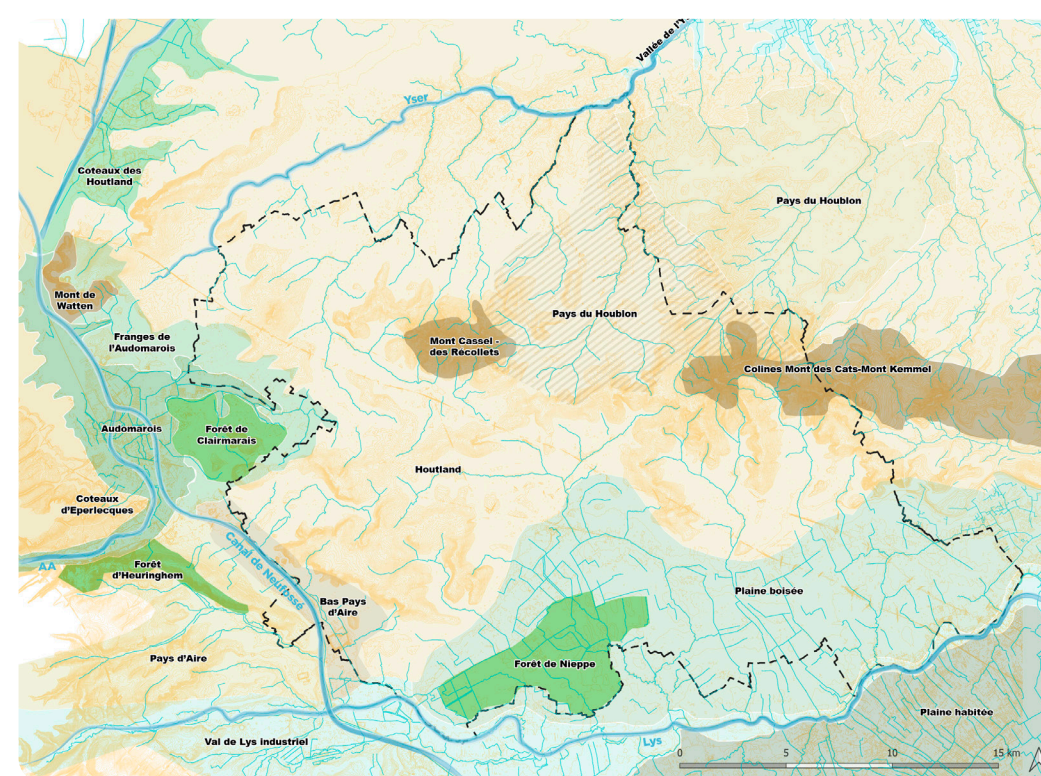
■ Carte des paysages
