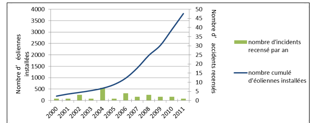
Figure 15 : Evolution du nombre d'incidents annuels en France et nombre d'éoliennes installées
