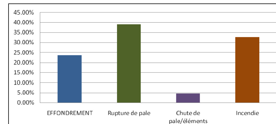
Figure 11 : Répartition des événements accidentels et de leurs causes premières dans le monde entre 2000 et 2011 (Source : CWIF)
