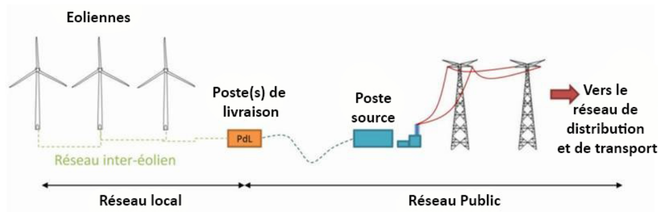
Figure 9 : Schéma de raccordement électrique d'un parc éolien
