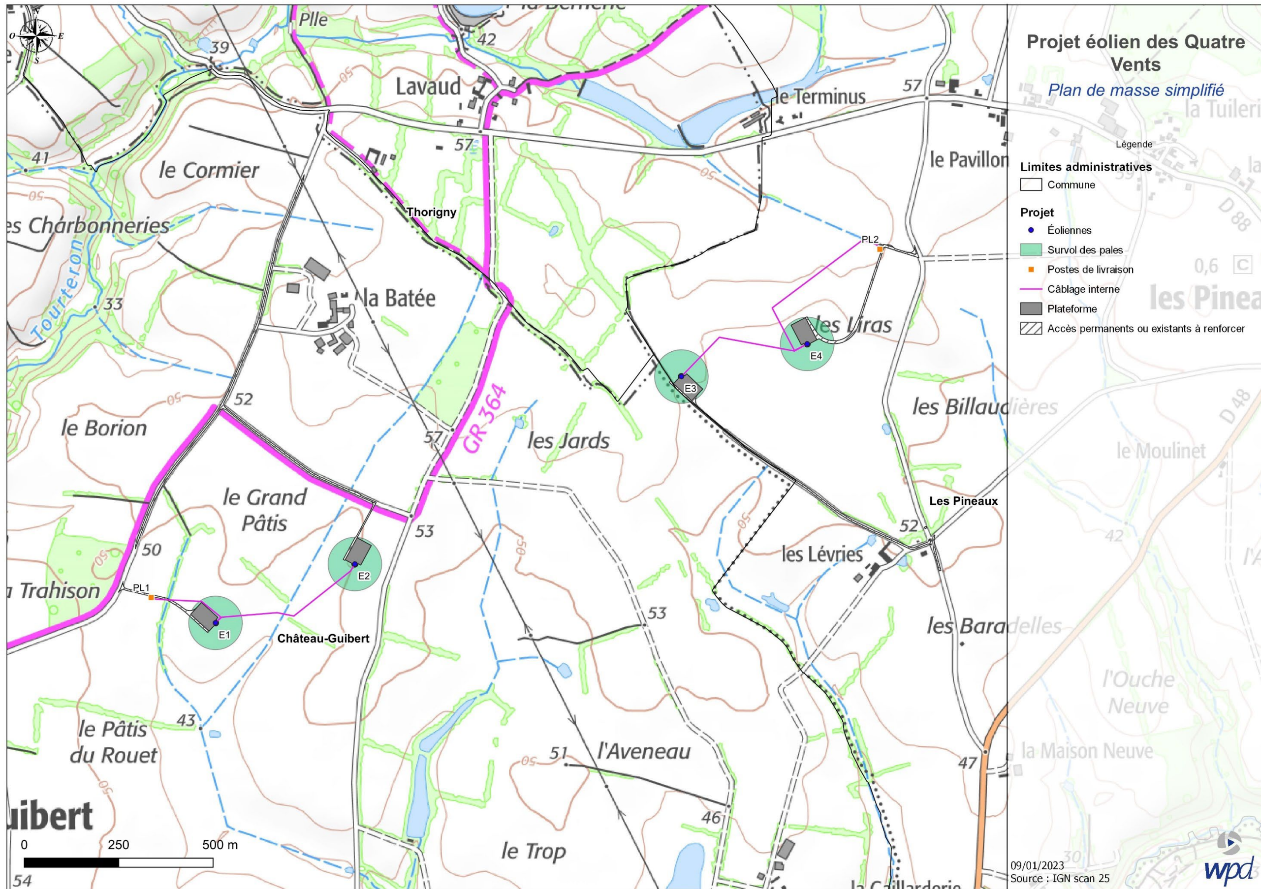
Carte 9 : Plan de masse du projet éolien des Quatre Vents
