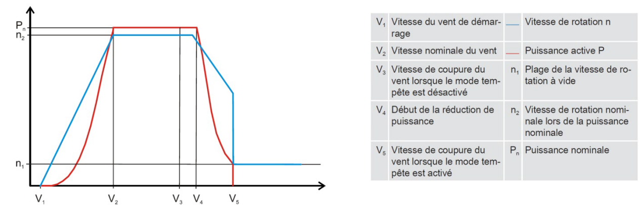
Figure 8 : Modes de fonctionnement : courbes de puissance en fonction de la vitesse du vent (Source : Guide technique, SER – FEE – INERIS)
