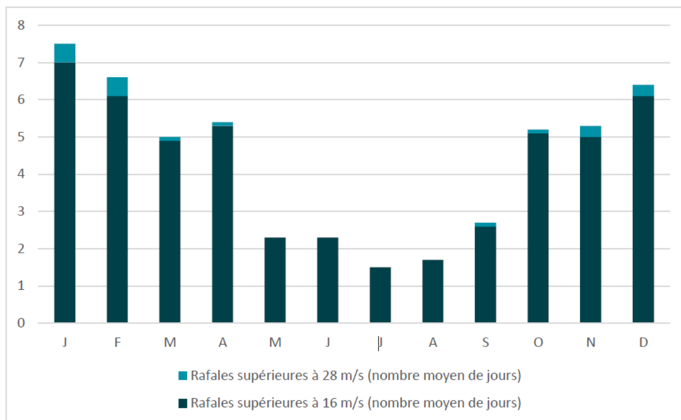
Figure 4 : Nombre moyen de jours avec des rafales de vents supérieures à 16 m/s (soit environ 57 km/h) et 28 m/s (soit environ 100
