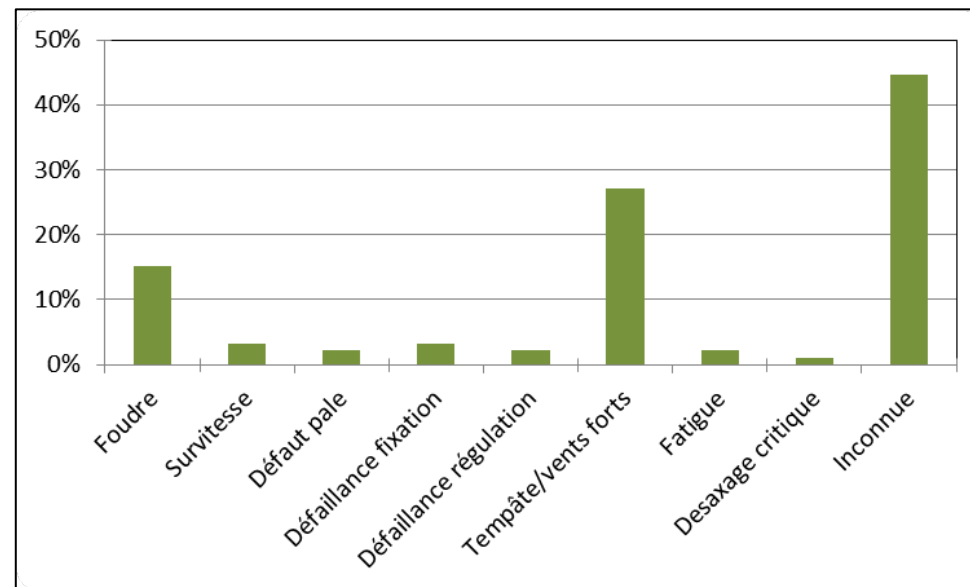
Figure 13 : Répartition des causes premières de rupture de pale (Source : CWIF)
