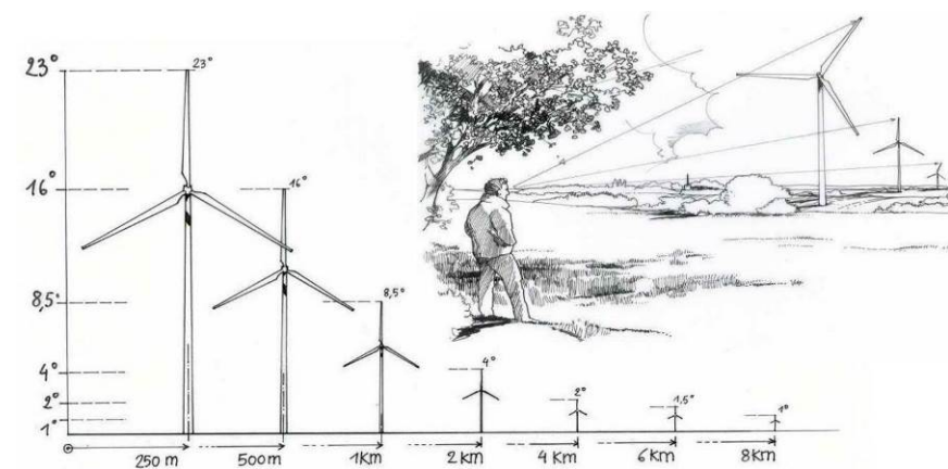
Illustration 124 : évolution de la perception de la hauteur d'une éolienne suivant la distance d'observation (source : guide relatif à l'élaboration des études d'impacts des projets de parcs éoliens terrestres - décembre 2016)
